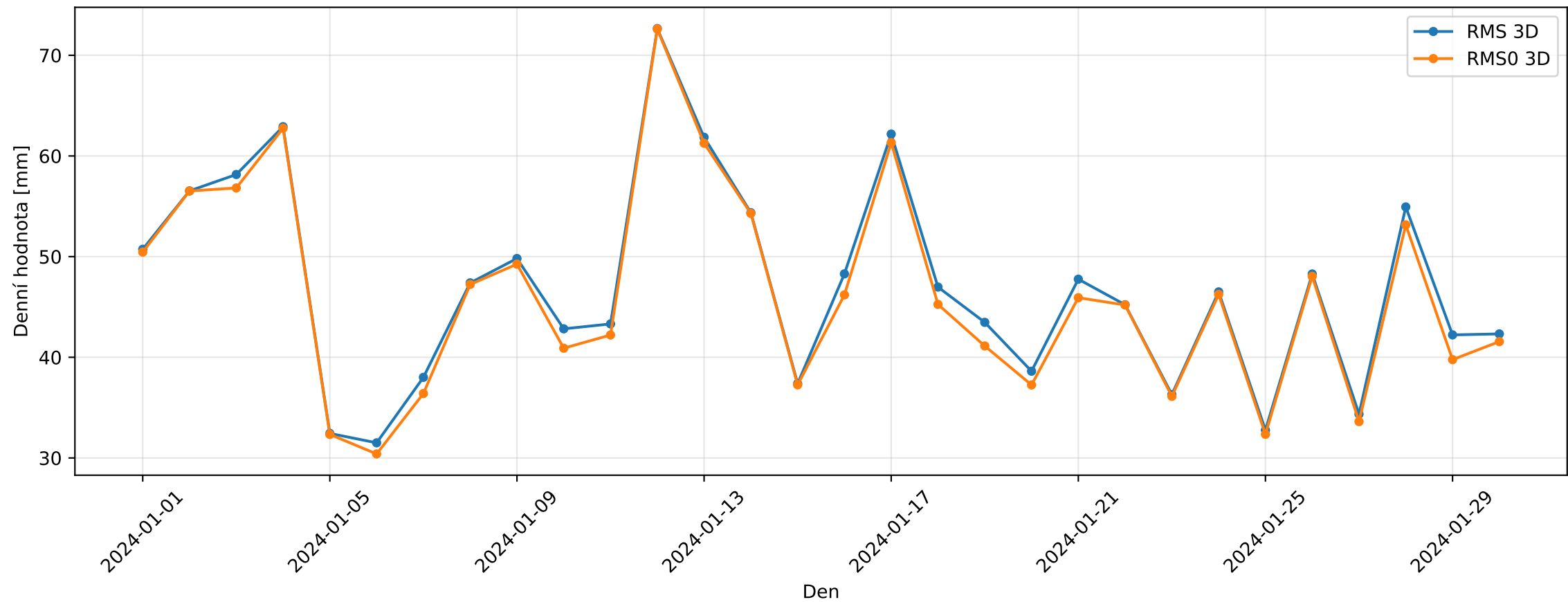
Porovnání RMS a RMS0 mezi GOP a SSA — H2C
