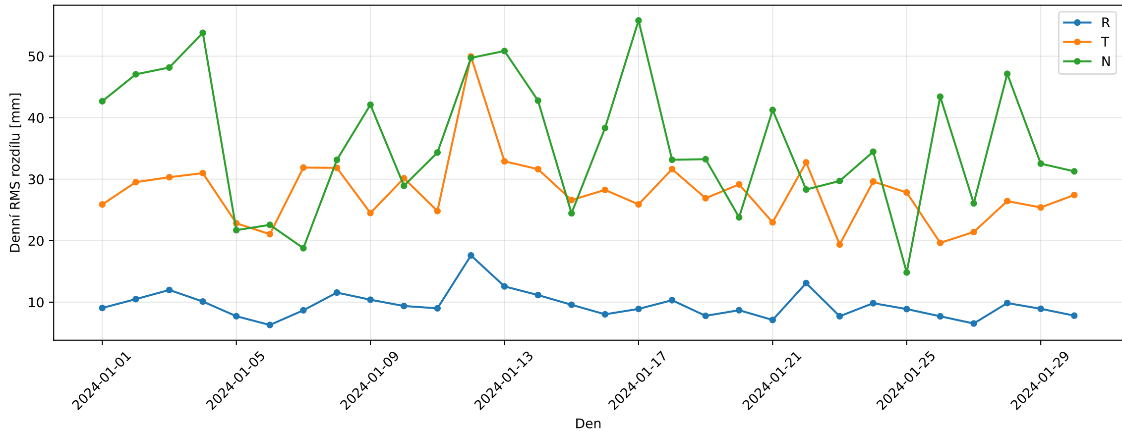
Denní RMS rozdílů mezi GOP a SSA v RTN — H2C
