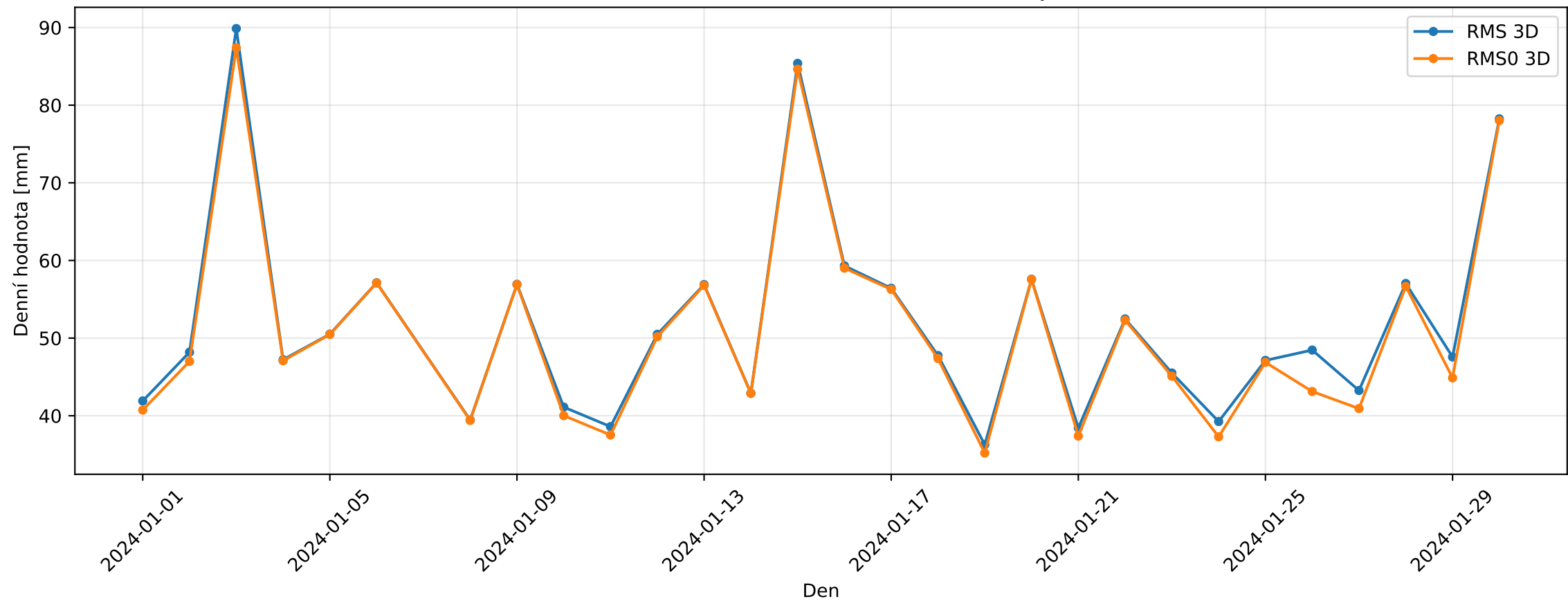
Porovnání RMS a RMS0 mezi GOP a SSA — JA3
