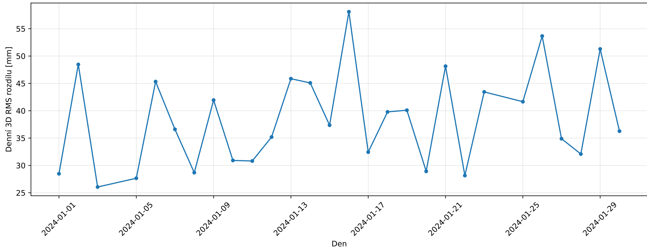
Denní 3D RMS rozdílů mezi GOP a SSA — S3A
