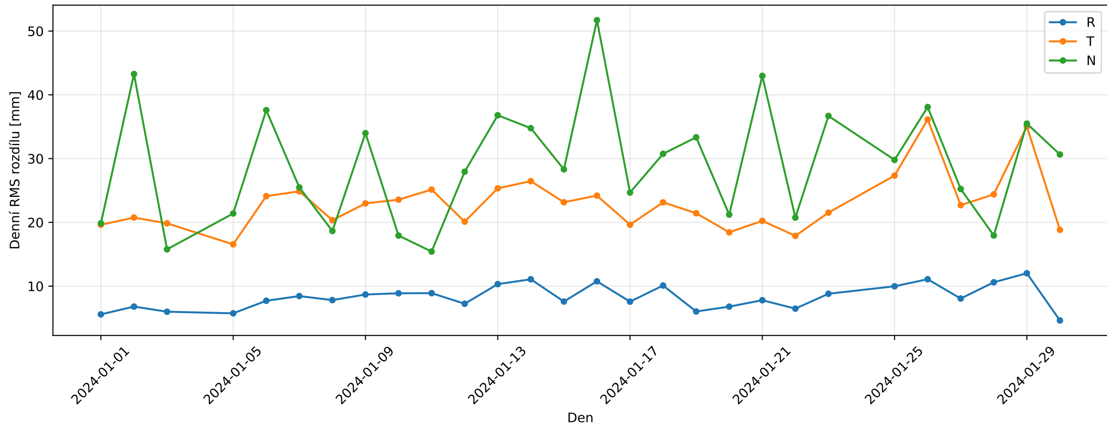
Denní RMS rozdílů mezi GOP a SSA v RTN — S3A
