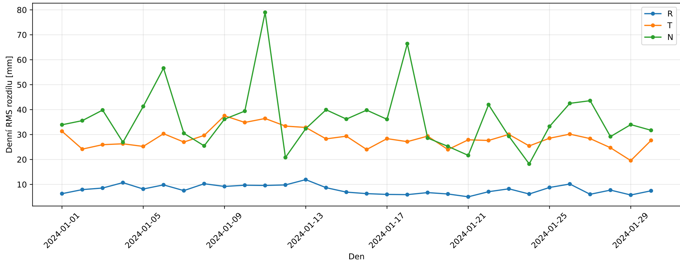
Denní RMS rozdílu mezi GOP a SSA v RTN — S6A
