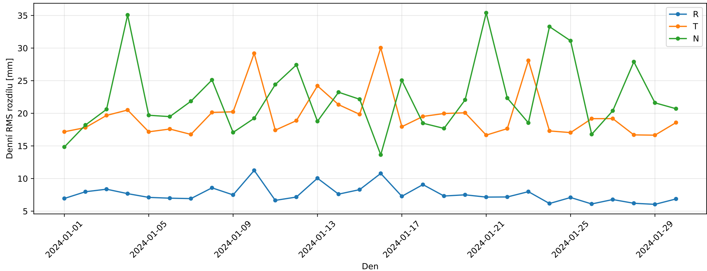
Denní RMS rozdílů mezi GOP a SSA v RTN — SRL
