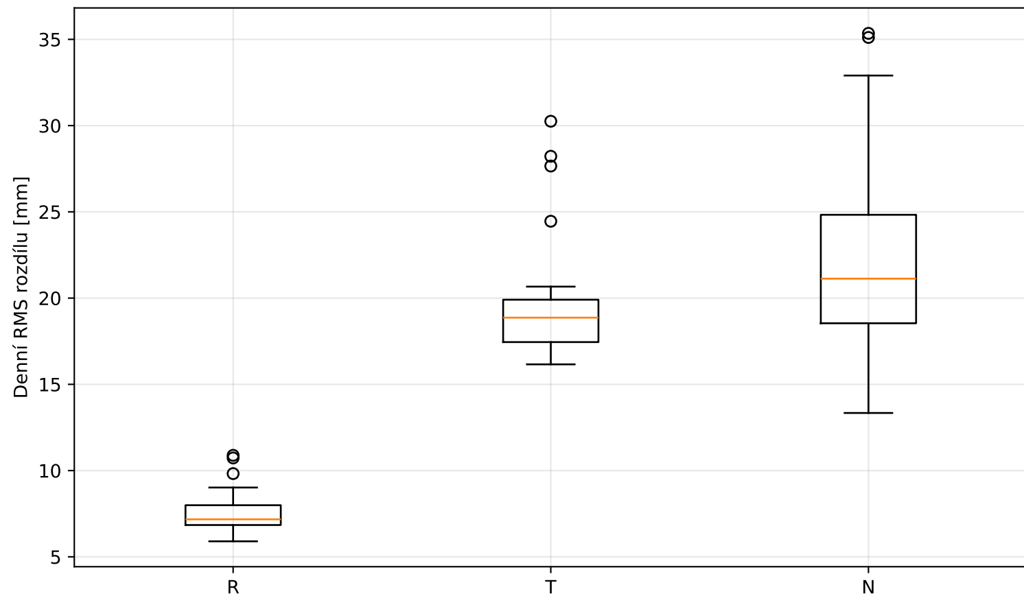
Rozdělení denních RMS rozdílů Bernese GOP-SSA — SRL
