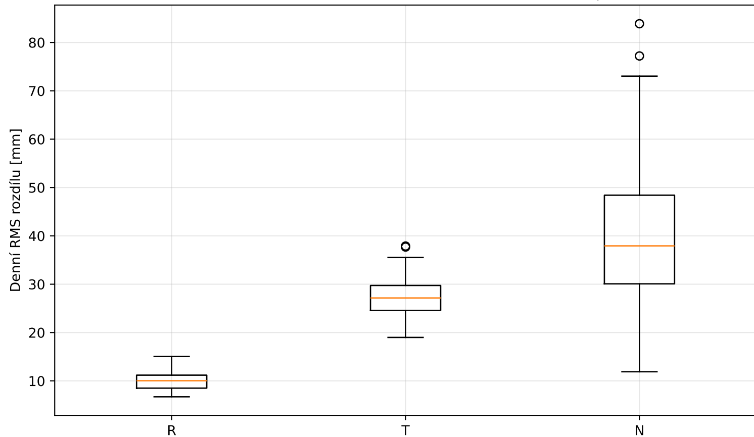
Rozdělení denních RMS rozdílů mezi GOP a SSA — JA3
