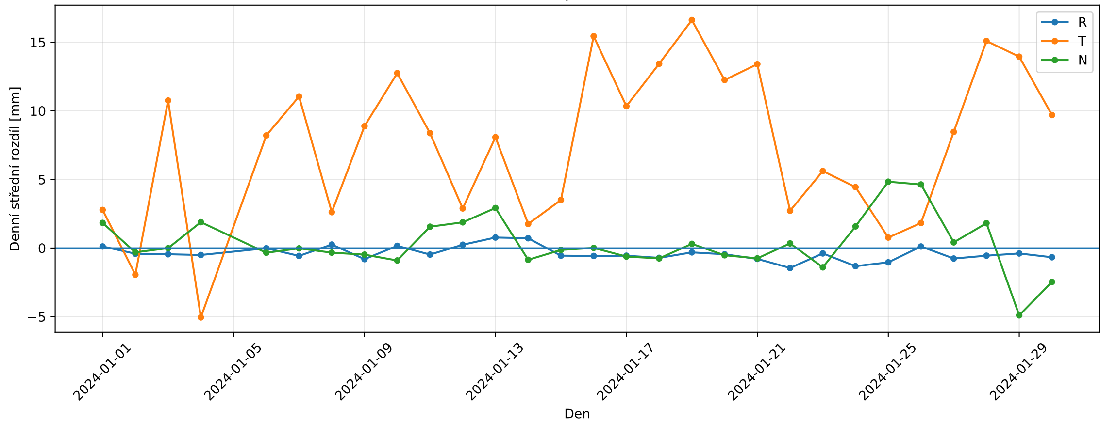
Denní střední rozdíly Bernese ZAZG v RTN
