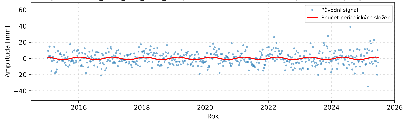
gop25wd04_stcd_licb_detr_weighte - dU - Rekonstruovaný periodický signál
