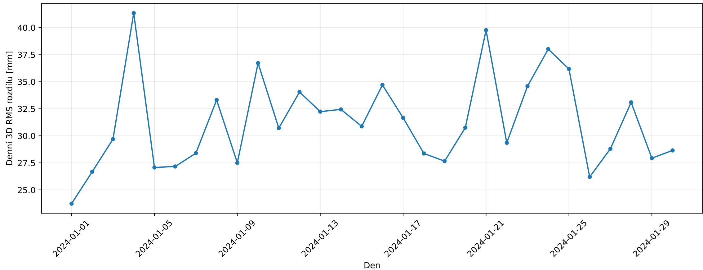
Denní 3D RMS rozdílů mezi GOP a SSA
