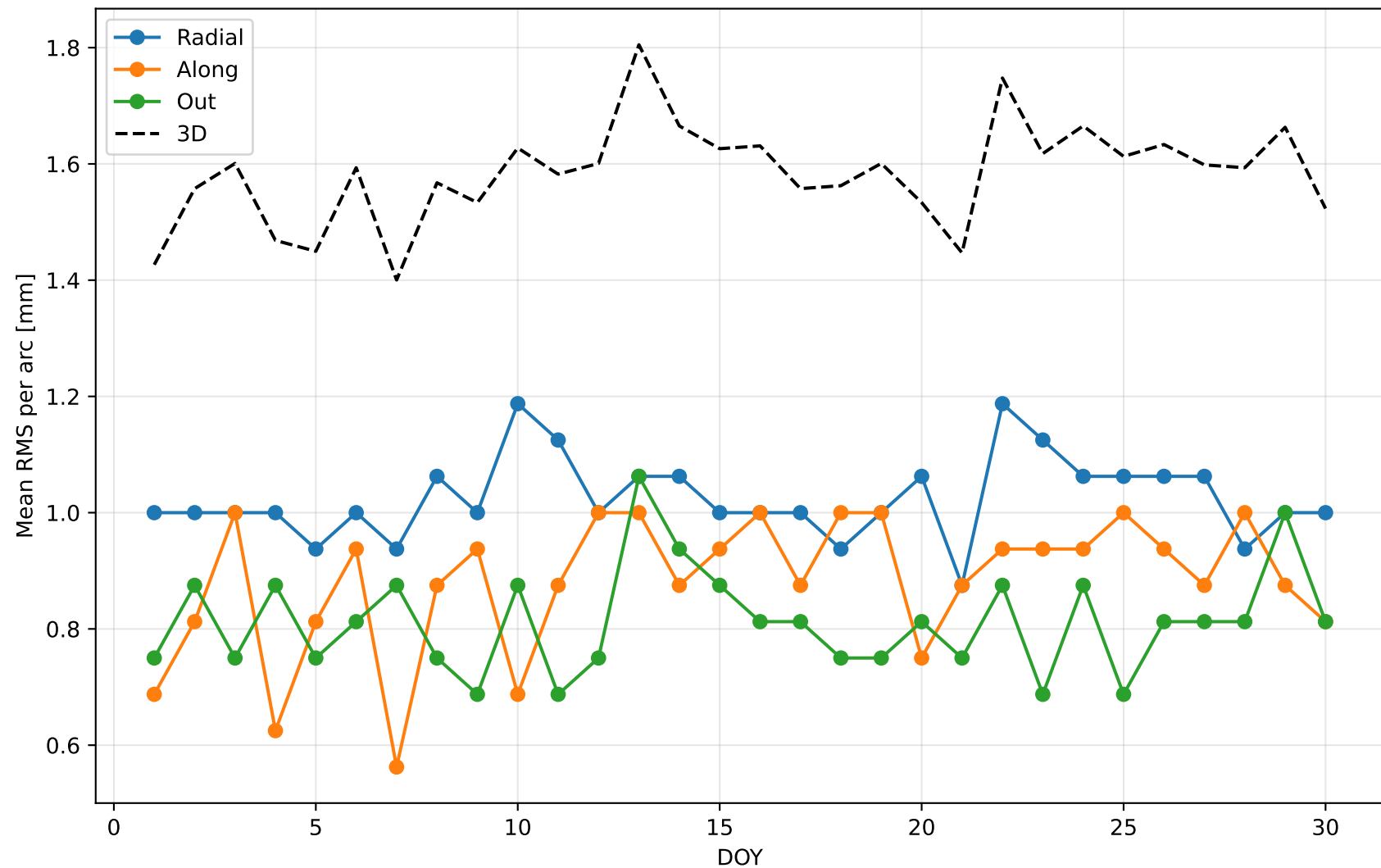
SA ZA: ORBGEN fit RMS, iteration 2
