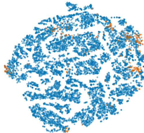
perplexity=100
