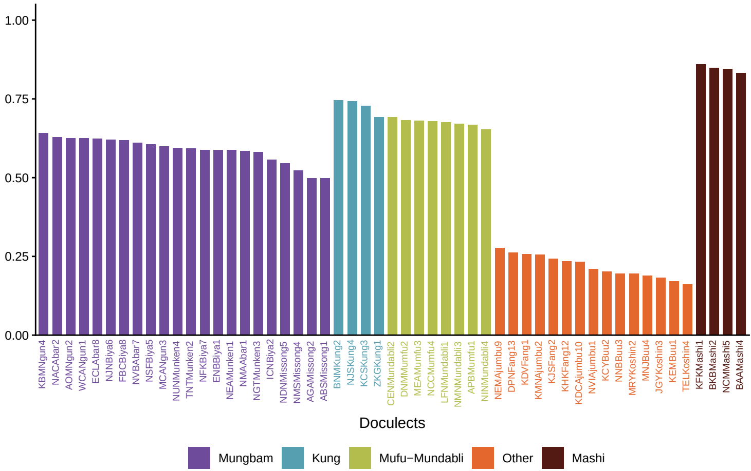
Silhouette width
