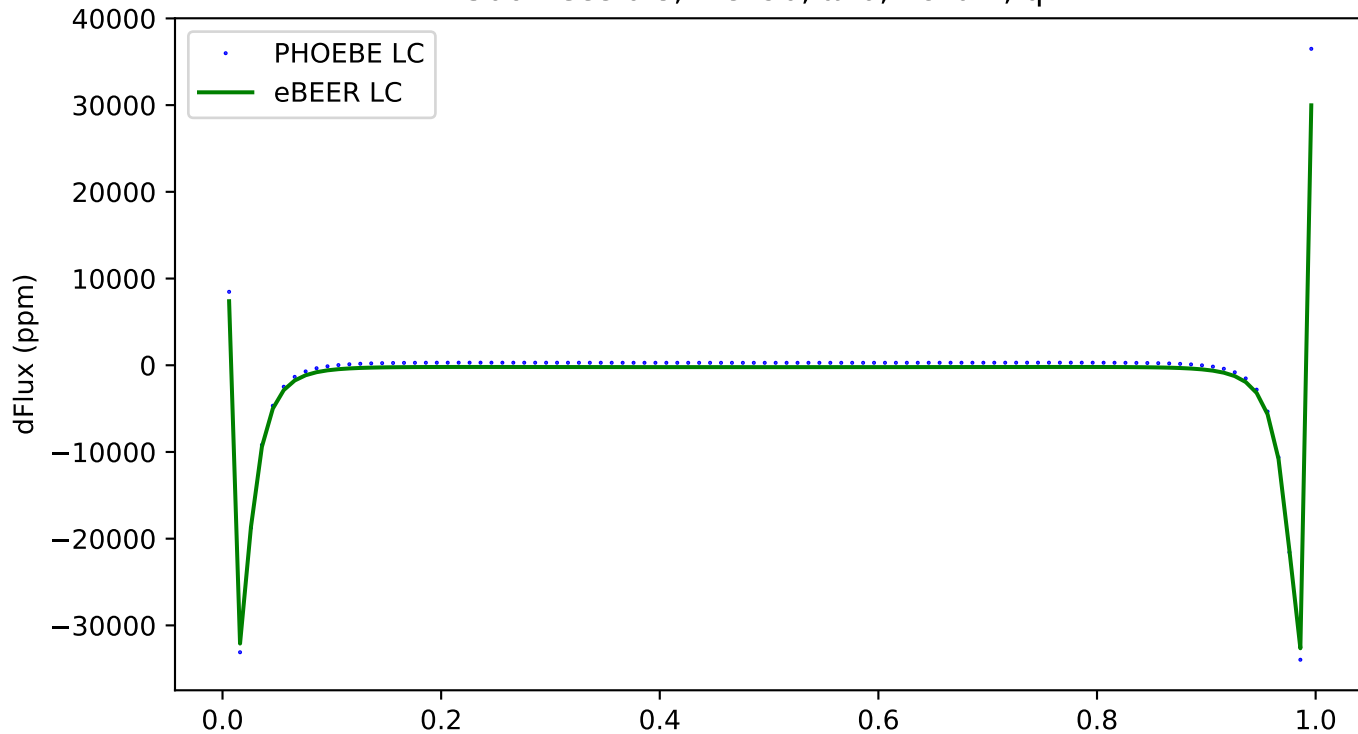
306 - ecc:0.8, incl:90, \omega :0, Porb:1, q:1
