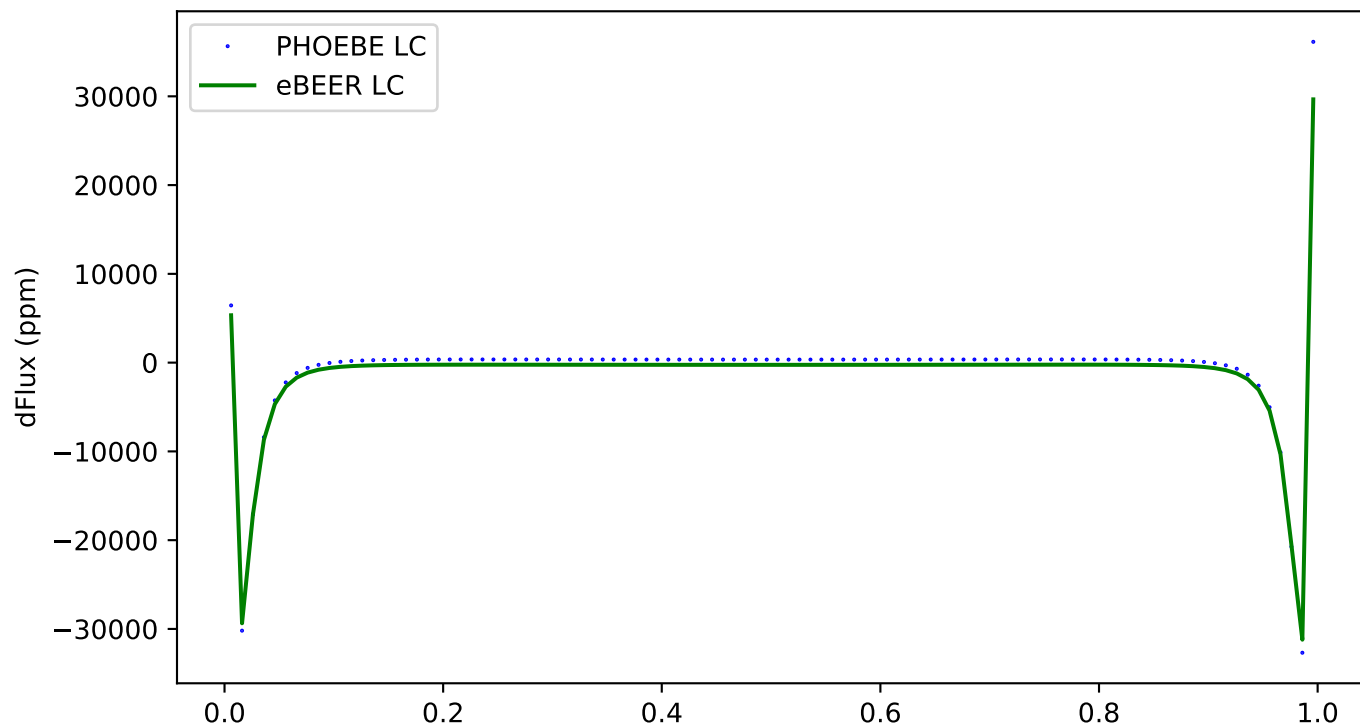
308 - ecc:0.8, incl:90, \omega :0, Porb:1, q:2
