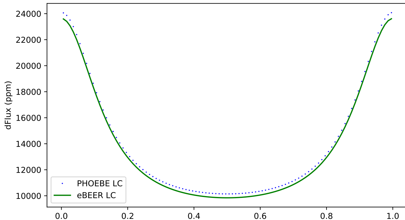
126 - ecc:0.3, incl:0, \omega :0, Porb:1, q:1
