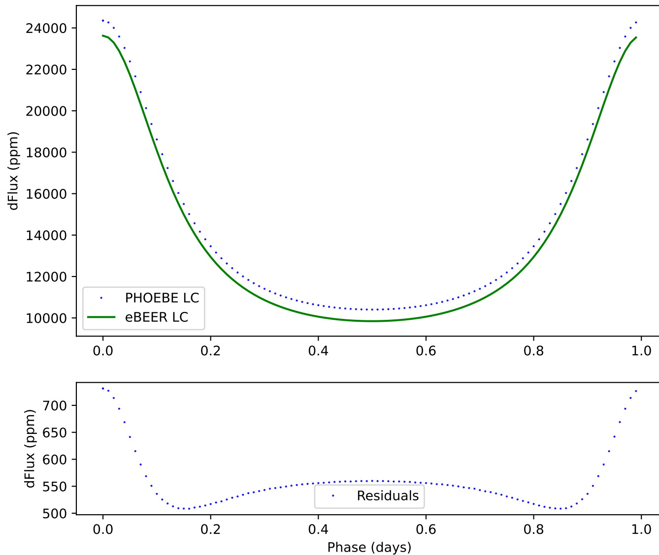
132 - ecc:0.3, incl:0, \omega :90, Porb:1, q:1
