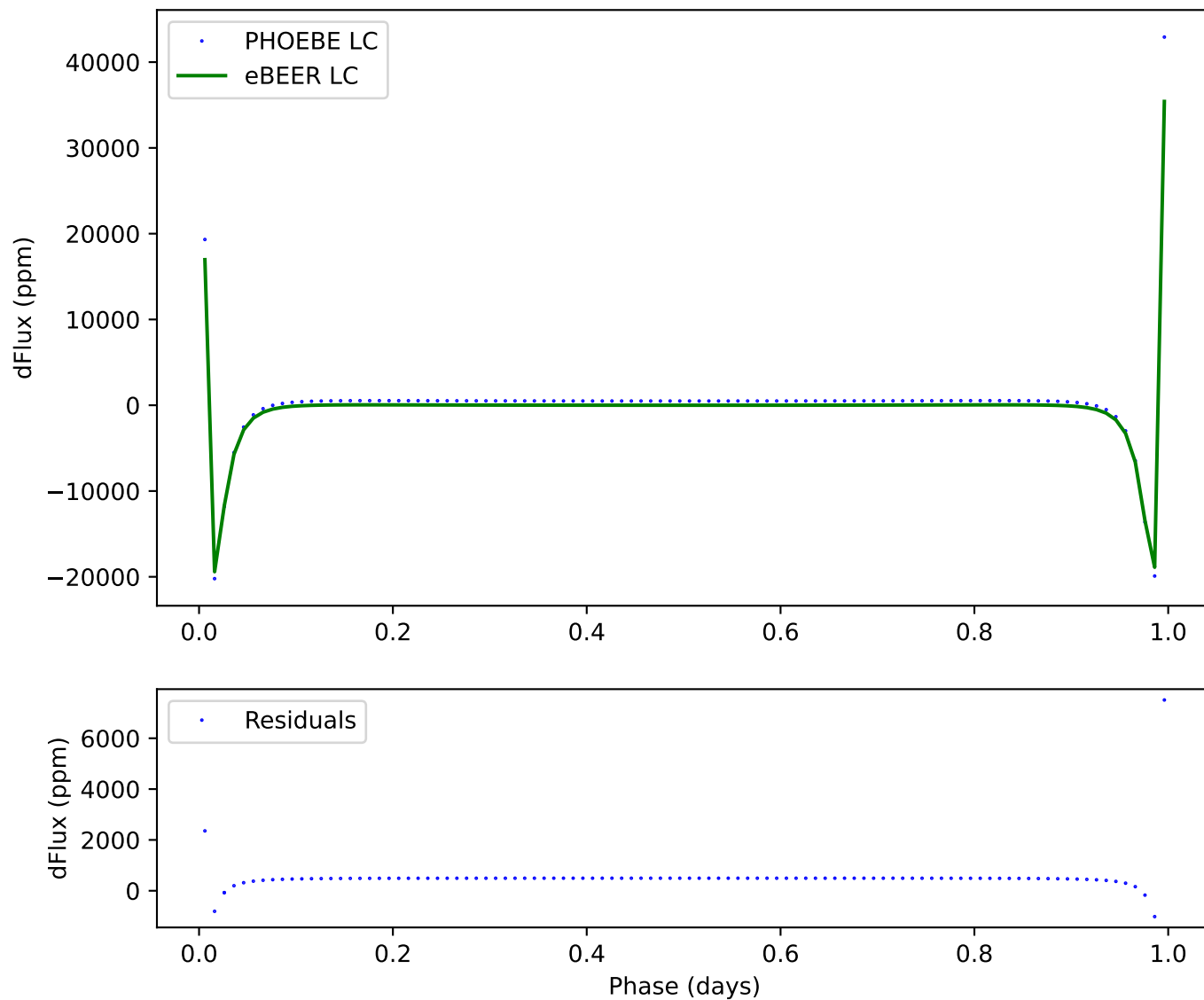
288 - ecc:0.8, incl:60, \omega :0, Porb:1, q:1
