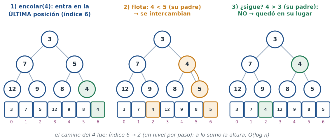
Figura 9.3: Encolar 4, paso a paso: entra en la última posición (índice 6), flota intercambiándose con su padre 5, y se detiene al encontrar un padre menor (3). Cada intercambio sube un nivel: O(\log n) .
