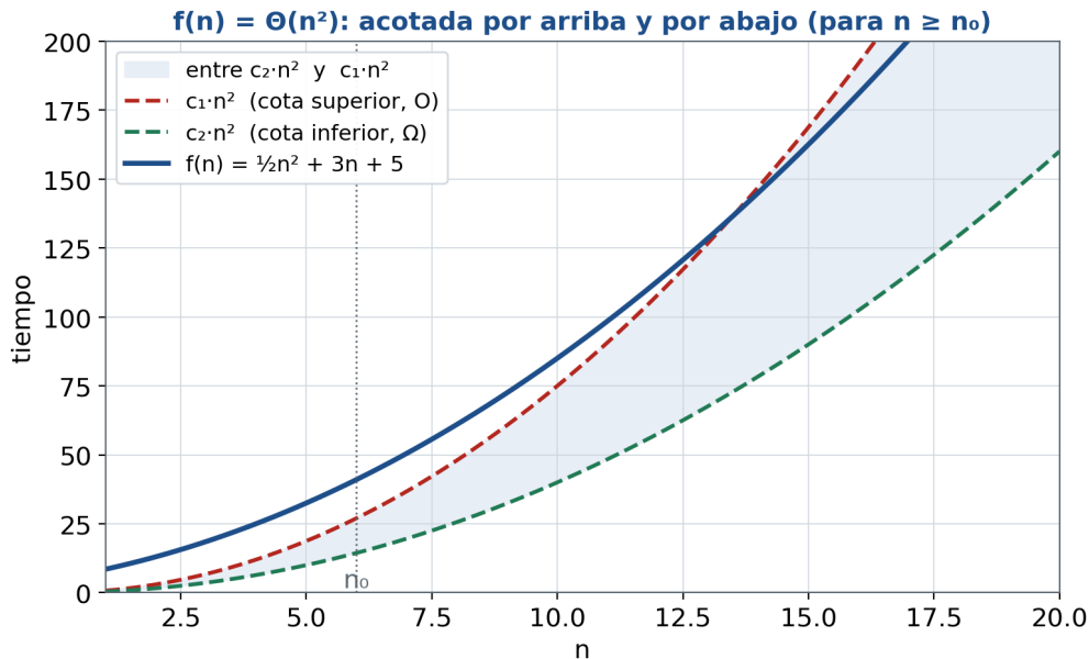
Figura 4.3: f(n) = \Theta(n^2) : queda “encajada” entre dos múltiplos de n^2 a partir de n_0 .
