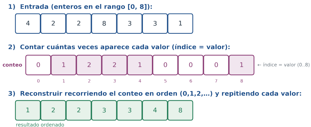
Figura 6.8: Counting sort paso a paso: (1) la entrada; (2) el arreglo de conteo, donde el índice es el valor y el contenido es la cantidad de apariciones; (3) la reconstrucción, recorriendo el conteo de 0 hacia arriba y escribiendo cada valor tantas veces como se contó.
