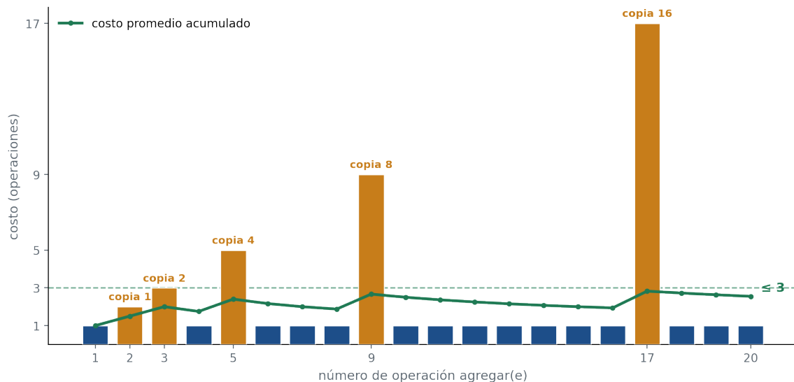
Figura 4.8: El costo de cada operación agregar con redimensión por duplicación. Casi todas cuestan 1 (azul); las que caen justo en una redimensión (naranja) pagan además la copia de todo lo existente. La línea verde —el promedio acumulado— nunca supera 3.
