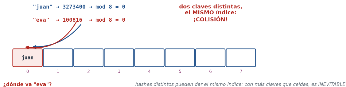
Figura 7.4: Una colisión real: "juan" y "eva" tienen hashCodes distintos (3273400 y 100816), pero ambos dan índice 0 en una tabla de 8 celdas. ¿Dónde va la segunda?
