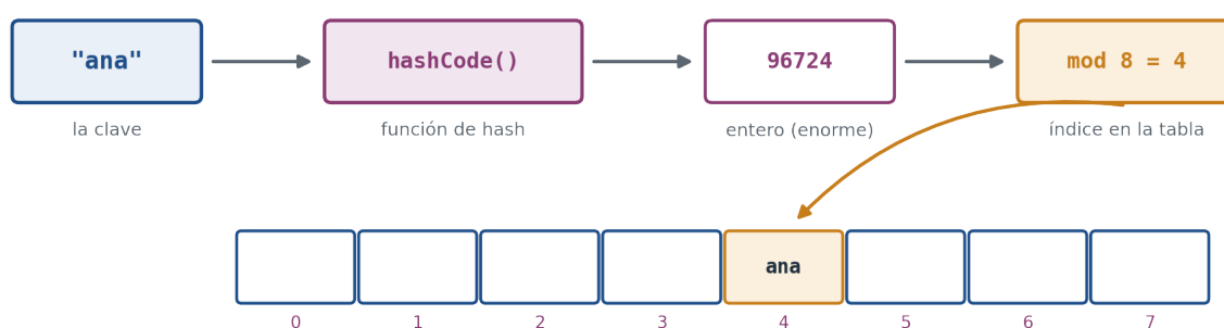
Figura 7.2: El camino de una clave hasta su celda: la función de hash la convierte en un entero (el hashCode() de Java), y el módulo lo lleva al rango de índices de la tabla. Para “ana”: hashCode 96724, y 96724 \bmod 8 = 4 .
