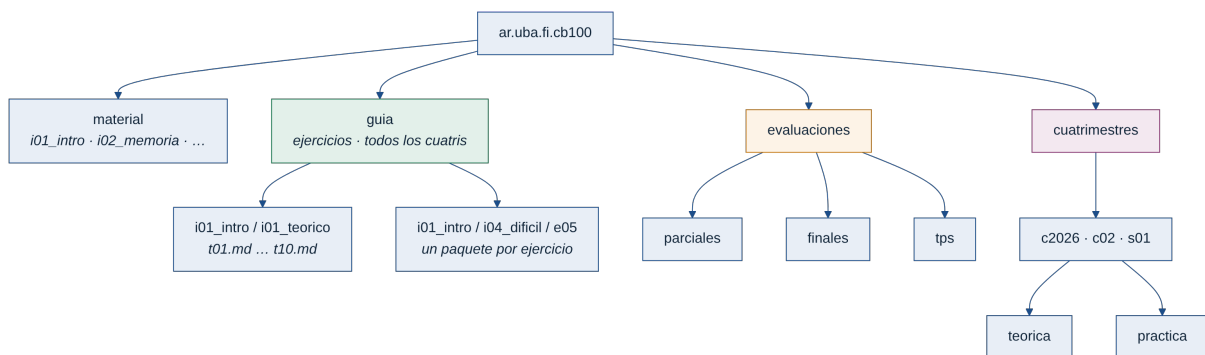
Figura 1B.20: Esquema de paquetes del repositorio único de la materia.
