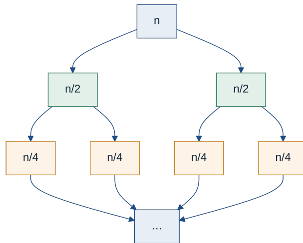
Figura 4.4: Árbol de recursión de T(n) = 2T(n/2) + n : cada nivel suma n ; hay \log_2 n niveles.
