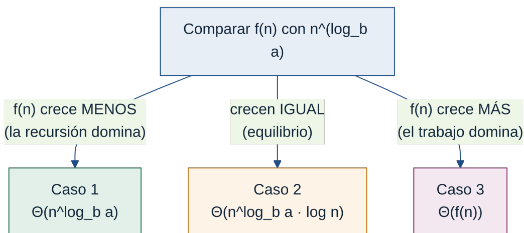
Figura 4.5: Los tres casos del Teorema Maestro según quién “gana” el crecimiento.
