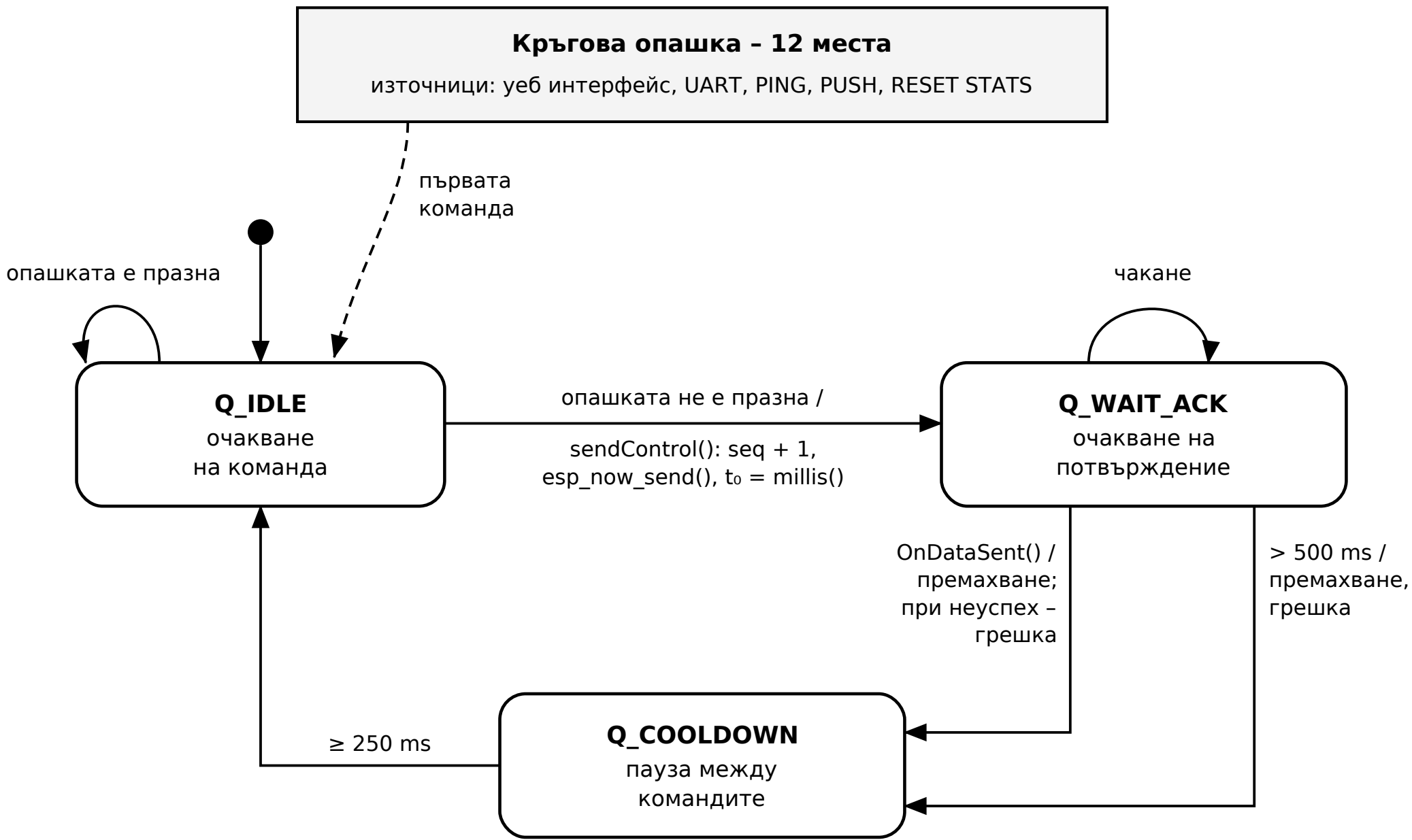
г) Краен автомат на опашката от команди
