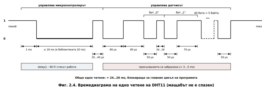
Фиг. 2.4. Времедиagramа на едно четене на DHT11 (машабът не е спазен)
