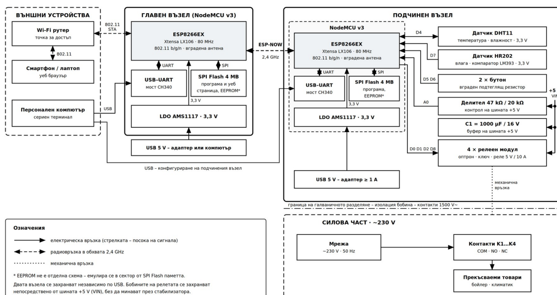
Фиг. 2.1. Блокова схема на хардуера
