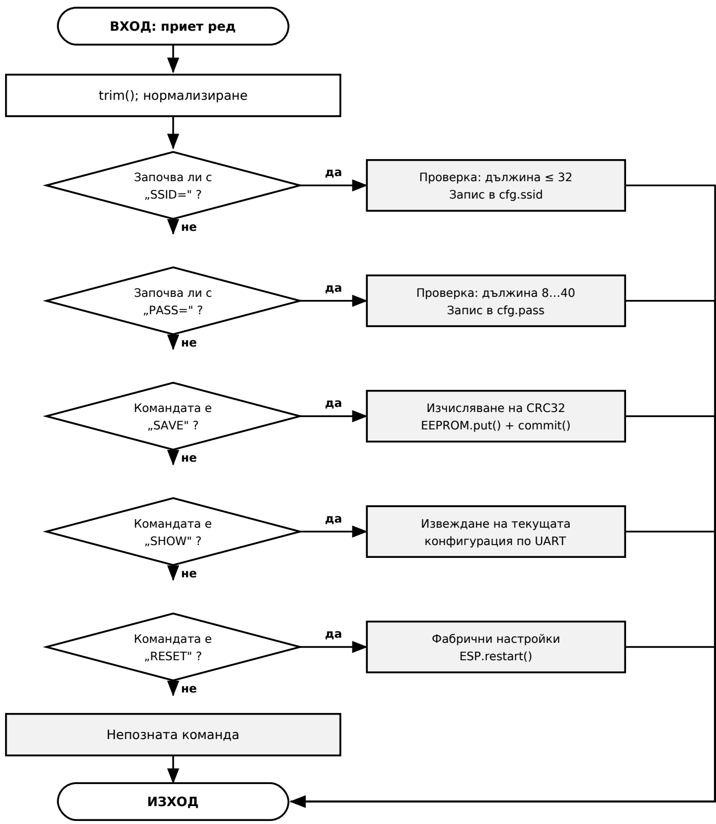
б) Алгоритъм за разбор на командите по UART
