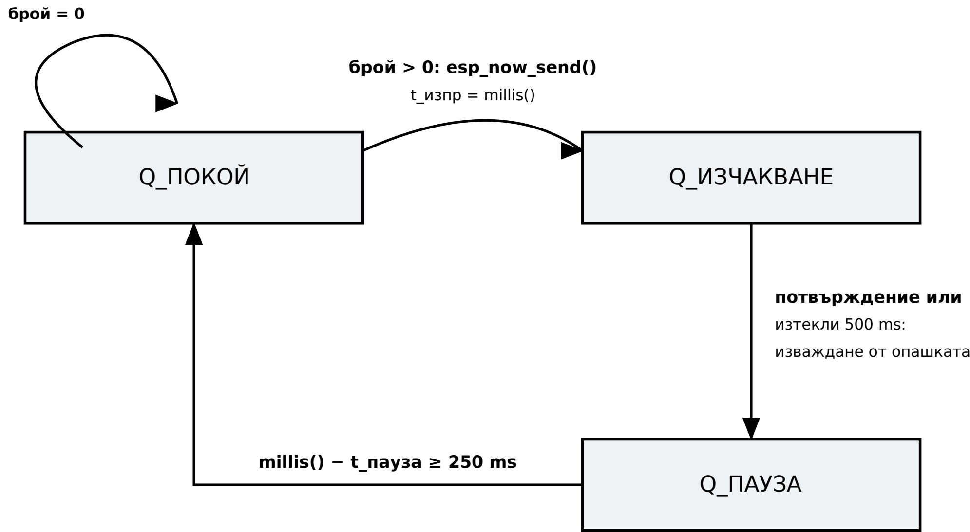
а) Алгоритъм на главния възел
