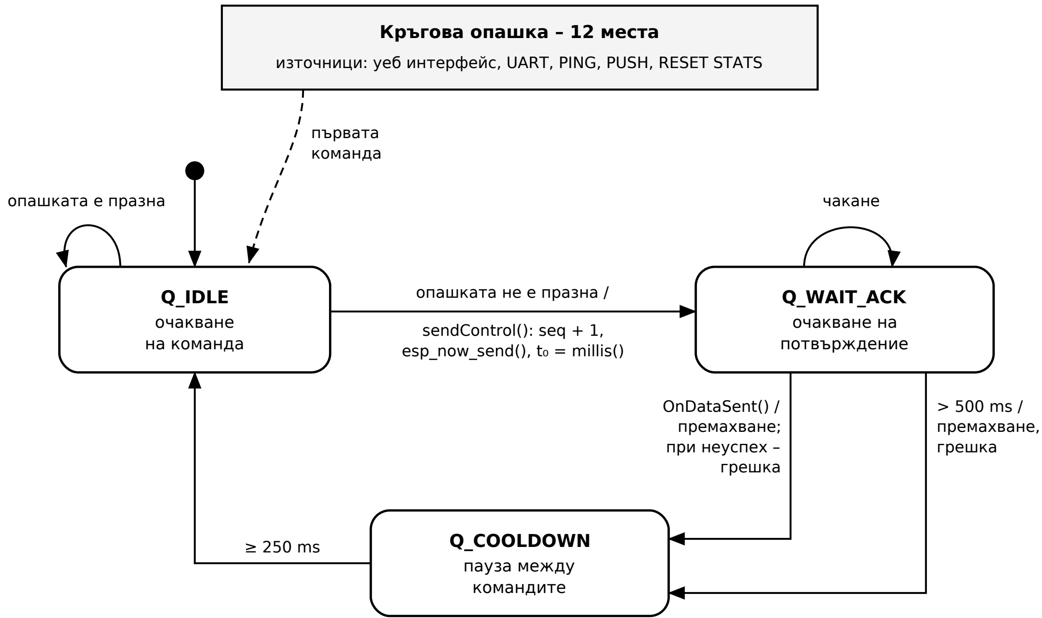
г) Краен автомат на опашката от команди
