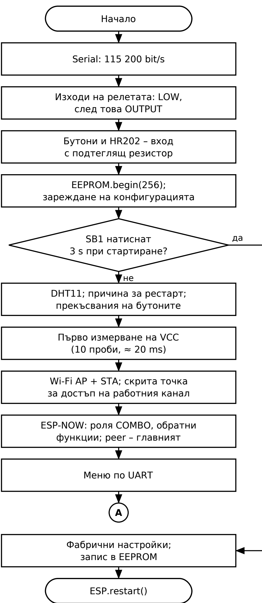
б) Алгоритъм на подчинения възел
