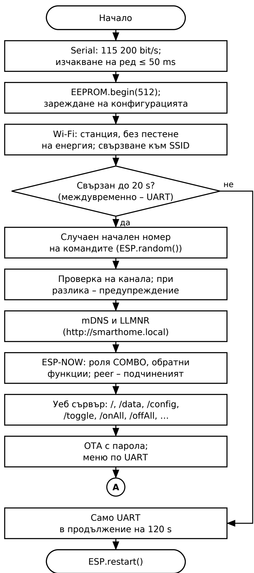
а) Алгоритъм на главния възел
