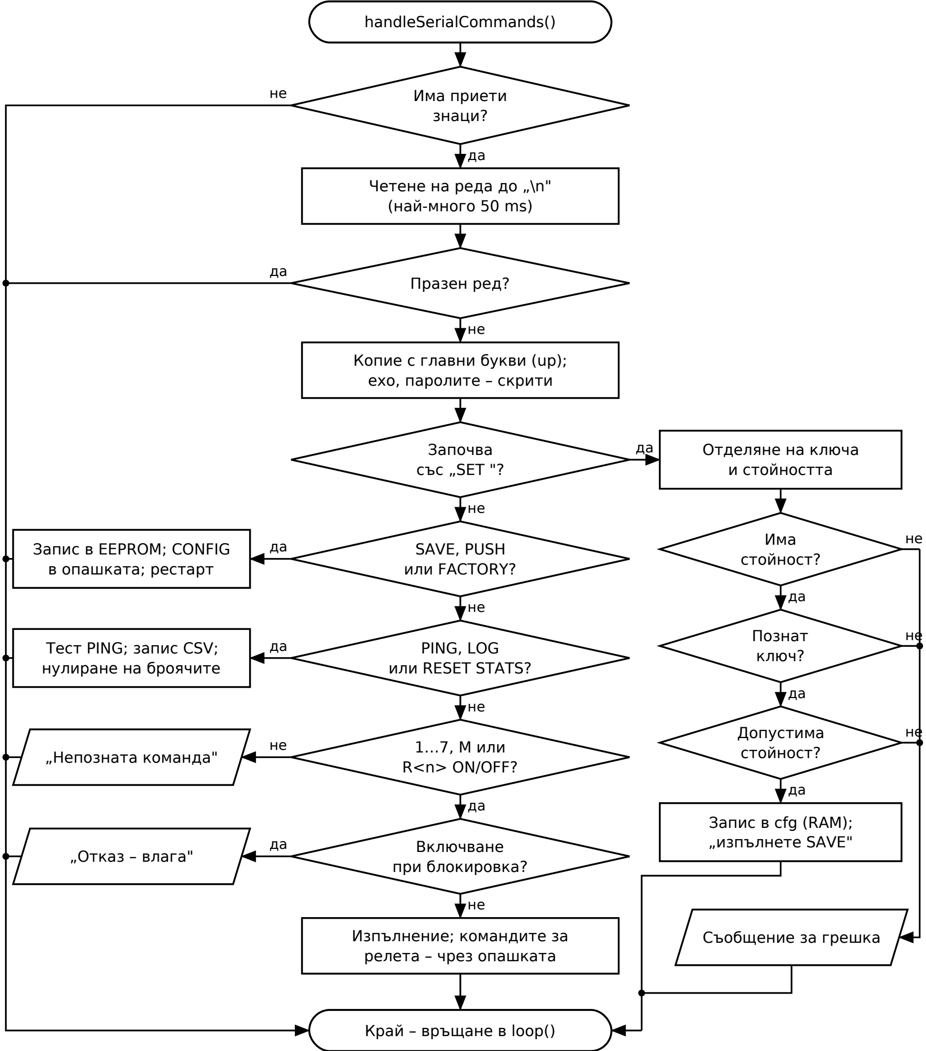
в) Обработка на командите по UART
