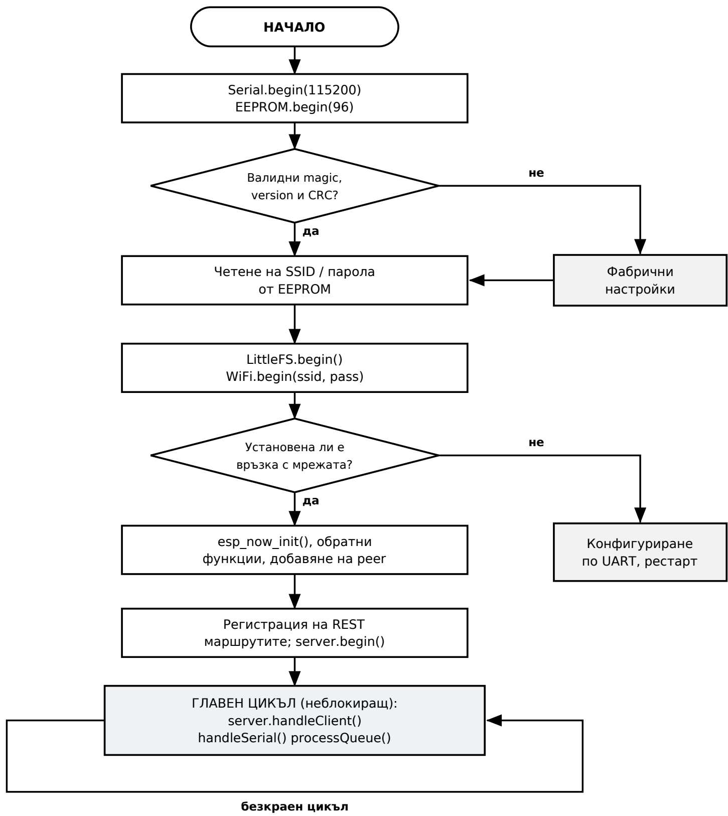
а) Алгоритъм на главния възел
