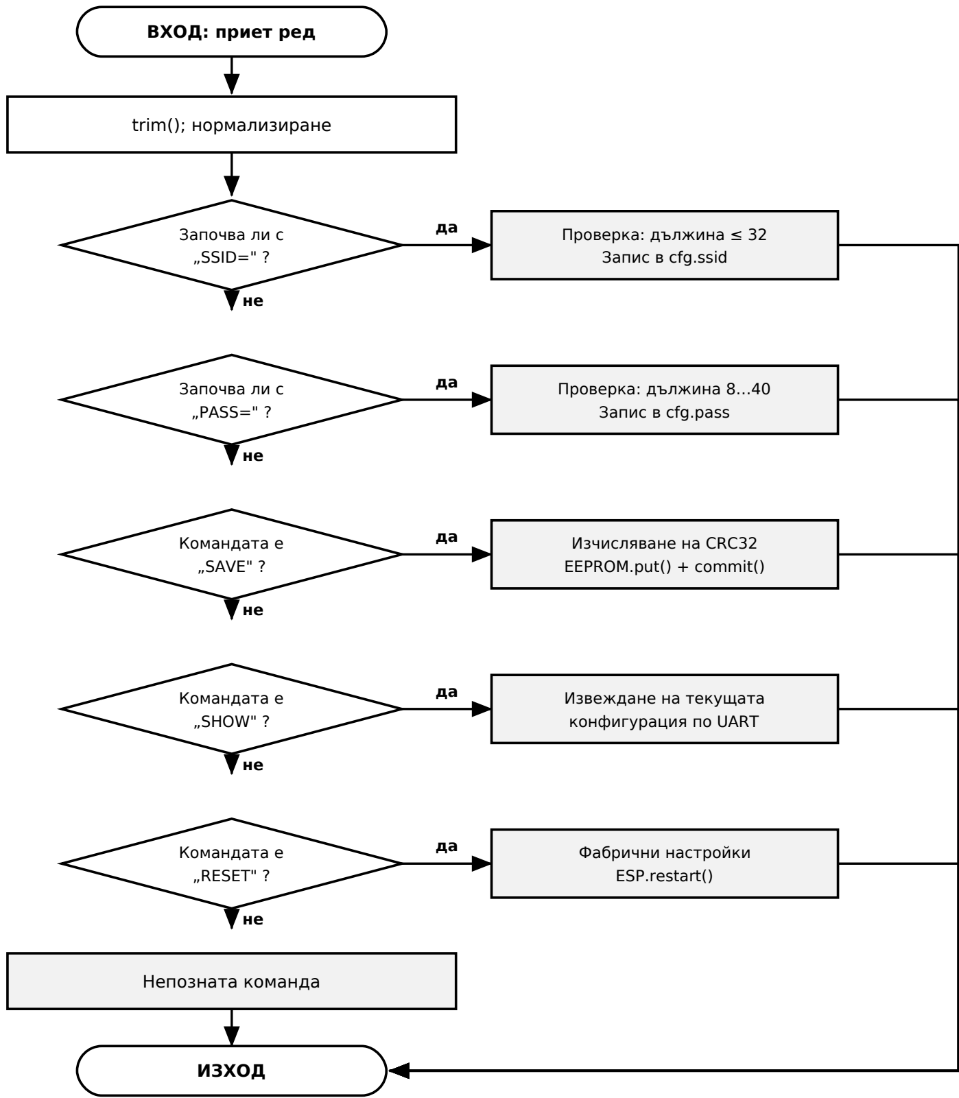
в) Разбор на командите по UART
