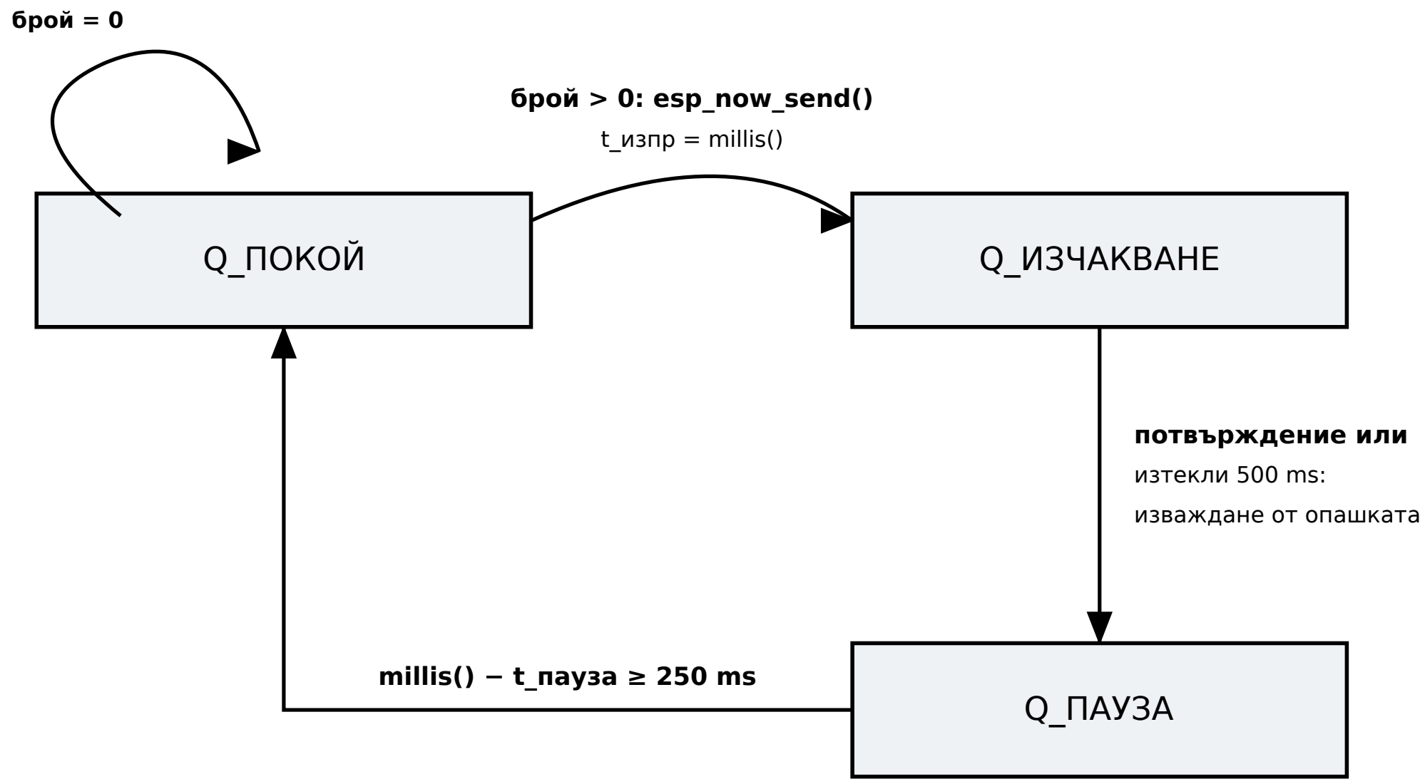
б) Алгоритъм на подчинения възел
