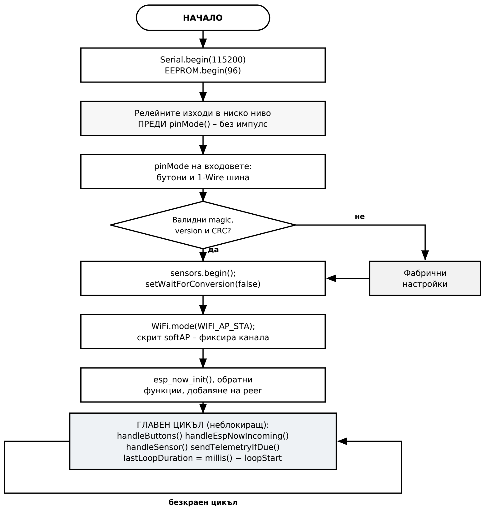
б) Алгоритъм на подчинения възел
