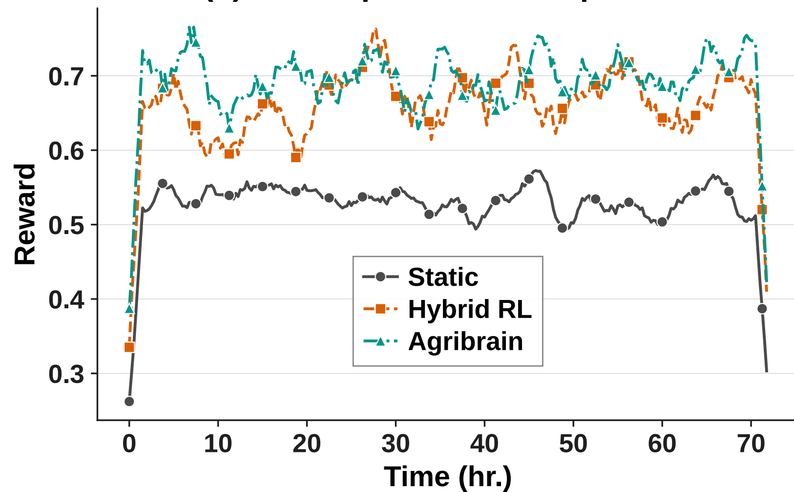
(d) Per-Step Reward Comparison
