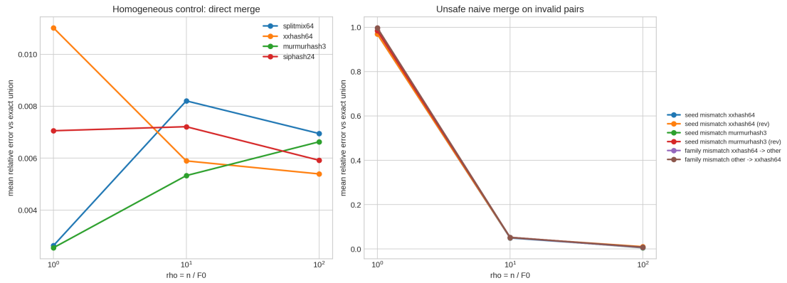
Figura 5.10: Esperimento di merge eterogeneo con funzioni di hash differenti
