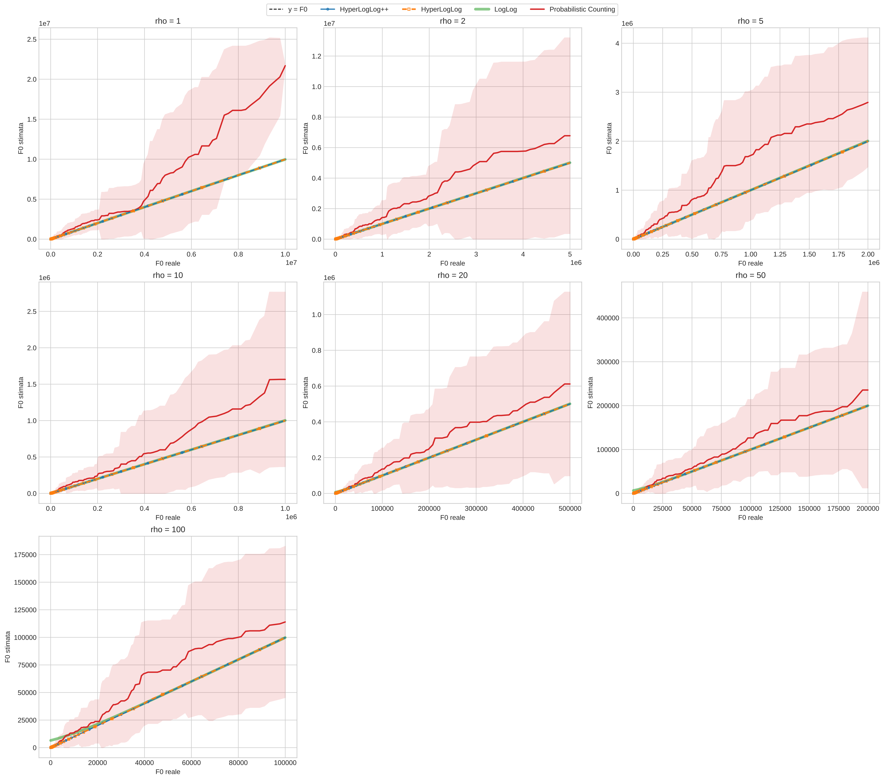
Cardinalità stimata rispetto alla cardinalità reale
