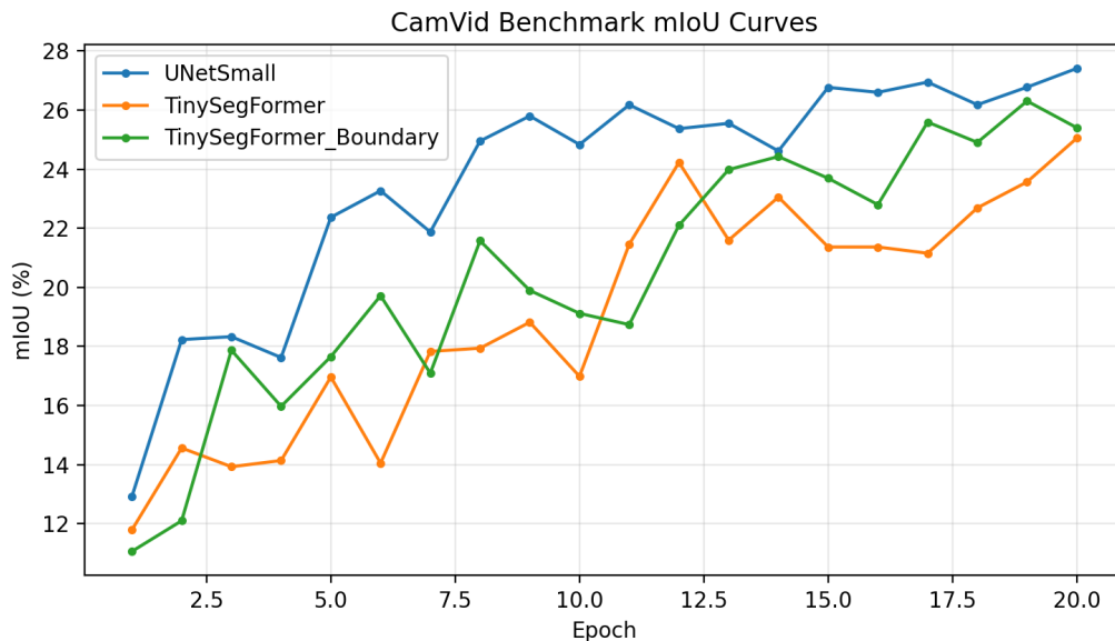
图 5 完整 CamVid 划分上不同方法的 mIoU 训练曲线
