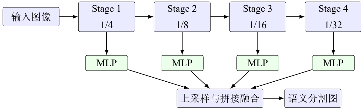
图 2 SegFormer 多尺度编码器与 MLP 解码器结构示意图
