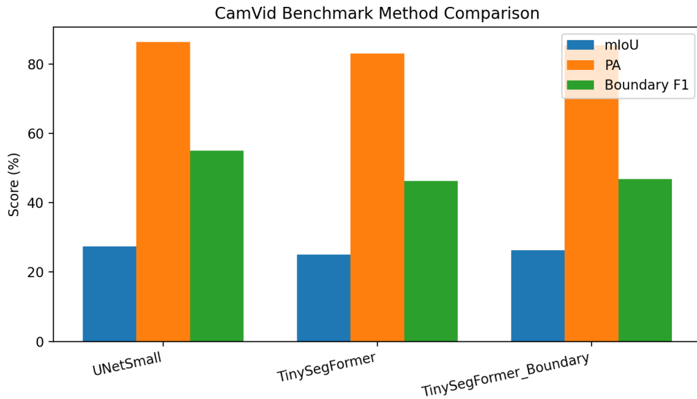
图 4 完整 CamVid 划分上的方法指标对比
