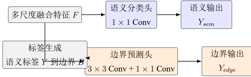
图 3 本文提出的边界增强 SegFormer 结构
