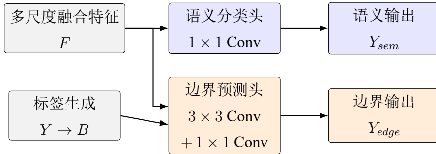
图 4 本文提出的边界增强 SegFormer 结构
