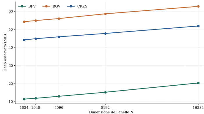
Figura 3.3: Heap osservato durante la creazione del contesto, con profondità 16.
