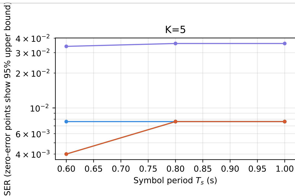
SER vs T_s ( N_{Tx} = 500 )
