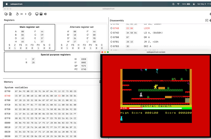
Slika 6.1: Posnetek zaslona emulatorja med izvajanjem igre Manic Miner.
