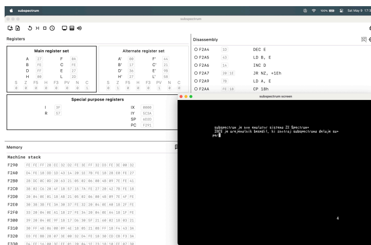
Slika 6.2: Posnetek zaslona emulatorja med izvajanjem urejevalnika besedil INES.
