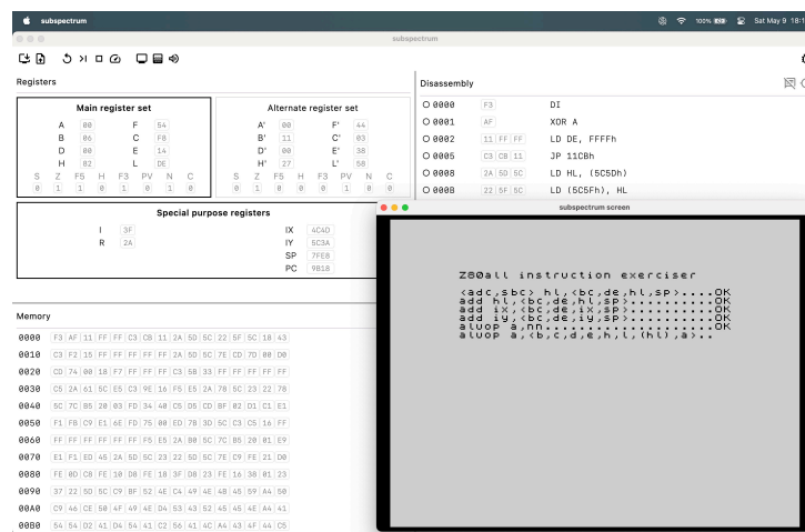
Slika 6.4: Posnetek zaslona emulatorja med izvajanjem testnega programa zexall.
