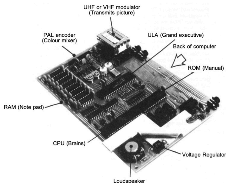
Slika 2.4: Skica notranjih komponent računalnika ZX Spectrum [21].
