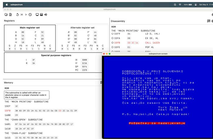
Slika 6.3: Posnetek zaslona emulatorja med izvajanjem igre Kontraband.
