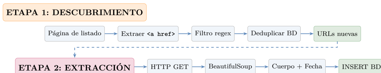
Figura 2: Pipeline de scraping en dos etapas: descubrimiento de URLs y extracción de contenido.
