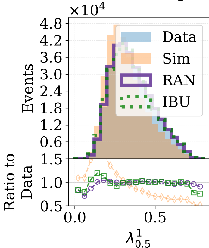
Les Houches Angularity
