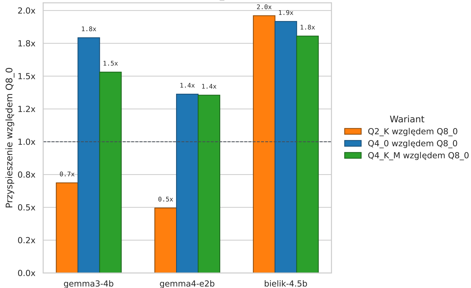
Przyspieszenie generacji względem Q8_0 (mediana modelu LN)
