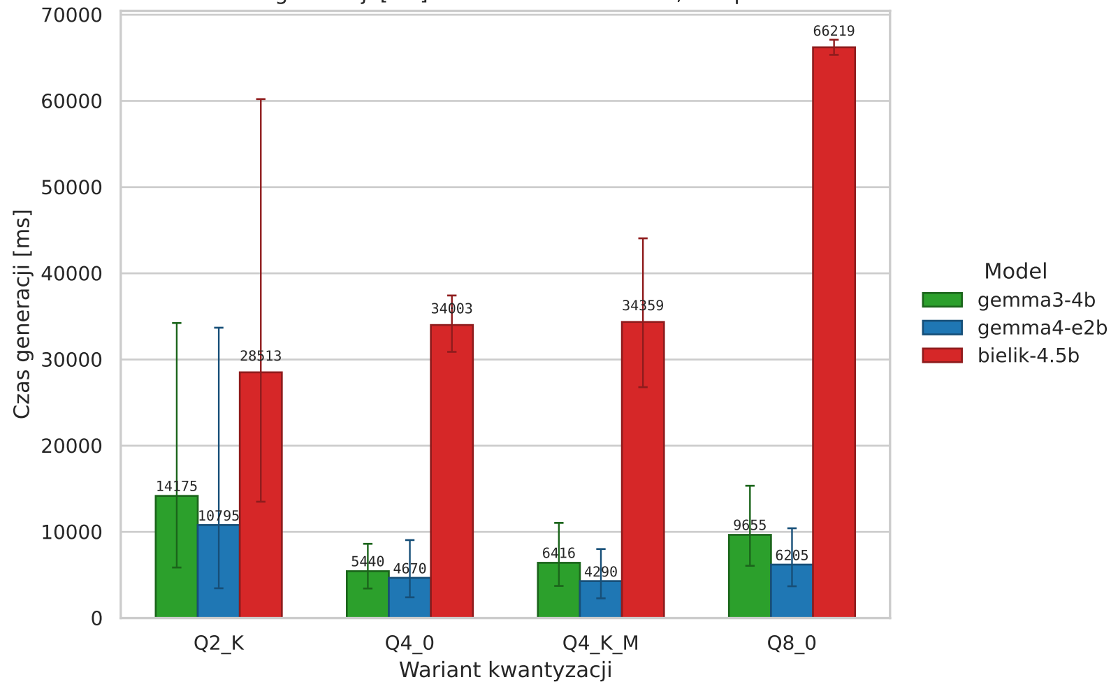
Czas generacji [ms] — mediana modelu LN, bez prefill
