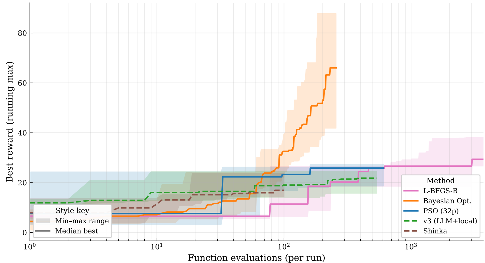
sw_011 — Maximise range proxy ( M \cdot L/D )
