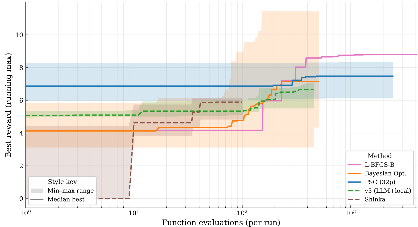
sw_014 — Maximise range proxy ( M \cdot L/D )
