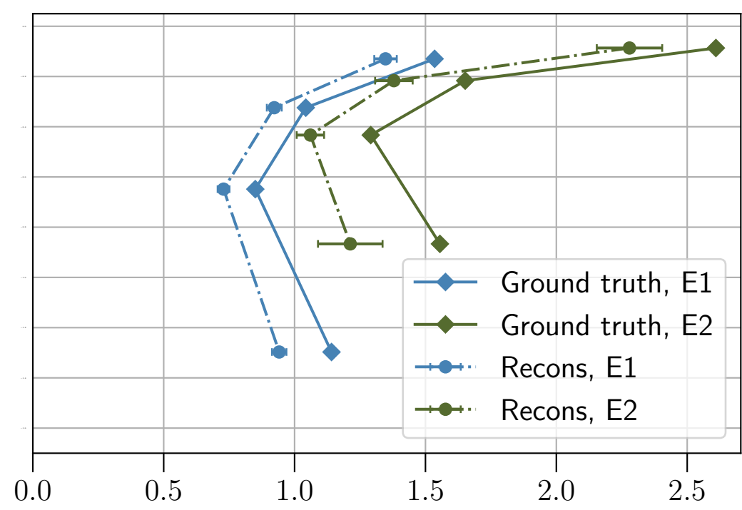
(b) \langle u_{RMS} \rangle , Cases E1 & E2
