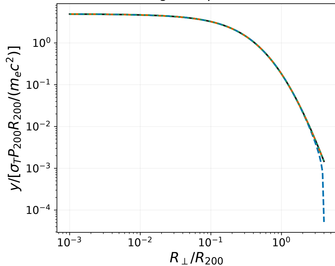
Battaglia12: \beta = 6.269
