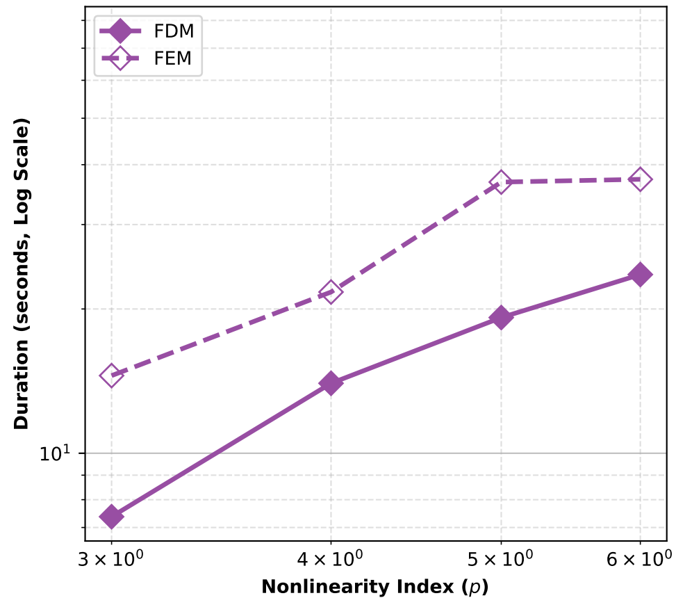
CVODE
