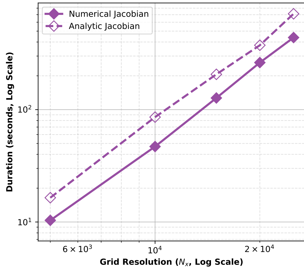
CVODE
