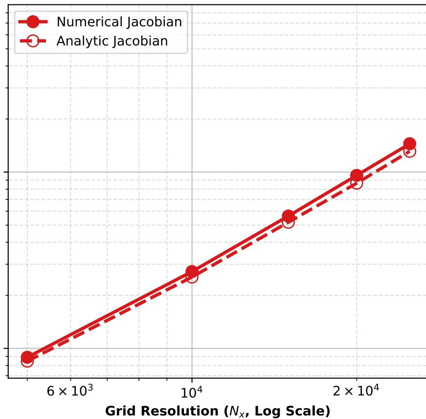
LSODA
