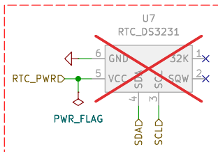
RTC_DS3231
