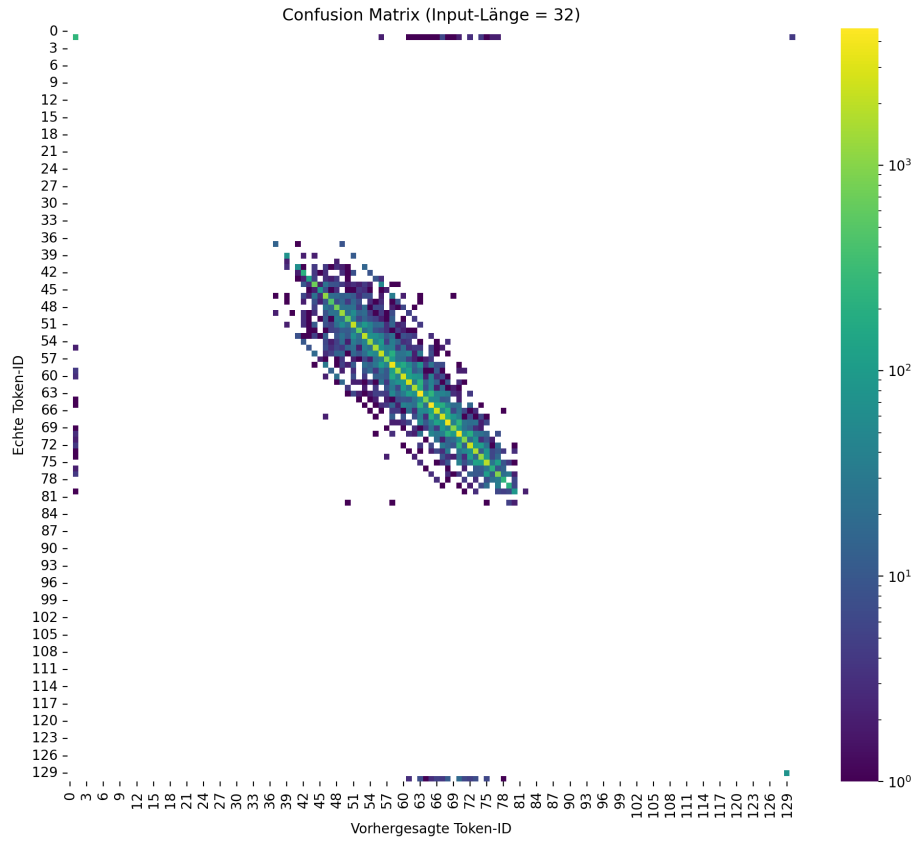
Figure 16: Confusion-Matrix, Input-Länge von 32
