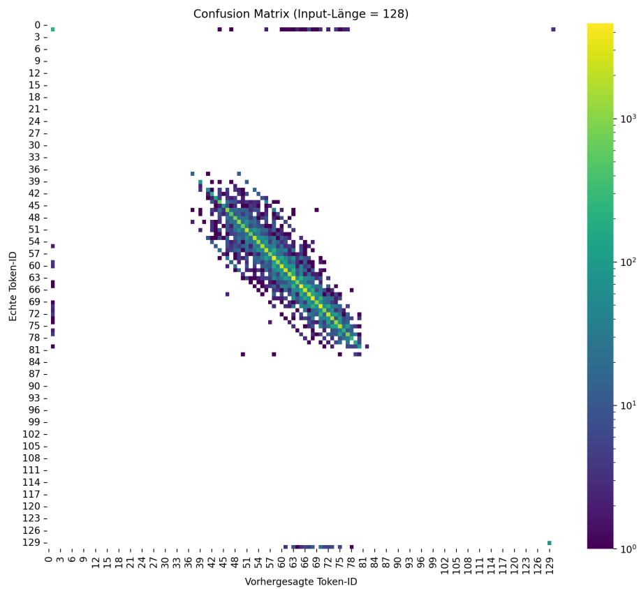
Figure 17: Confusion-Matrix, Input-Länge von 128
