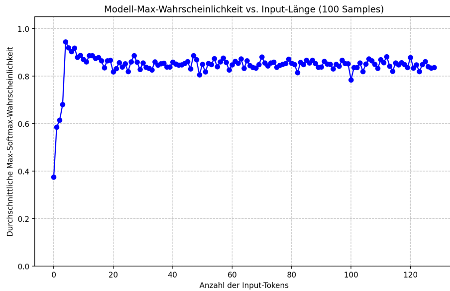
Figure 20: Maximale Wahrscheinlichkeiten für den nächsten Token in Abhängigkeit der Input-Länge
