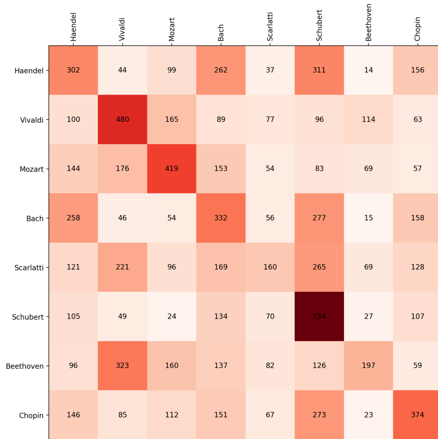
Figure 2: Klassifikation mit 1.000 Bäumen im Forest
