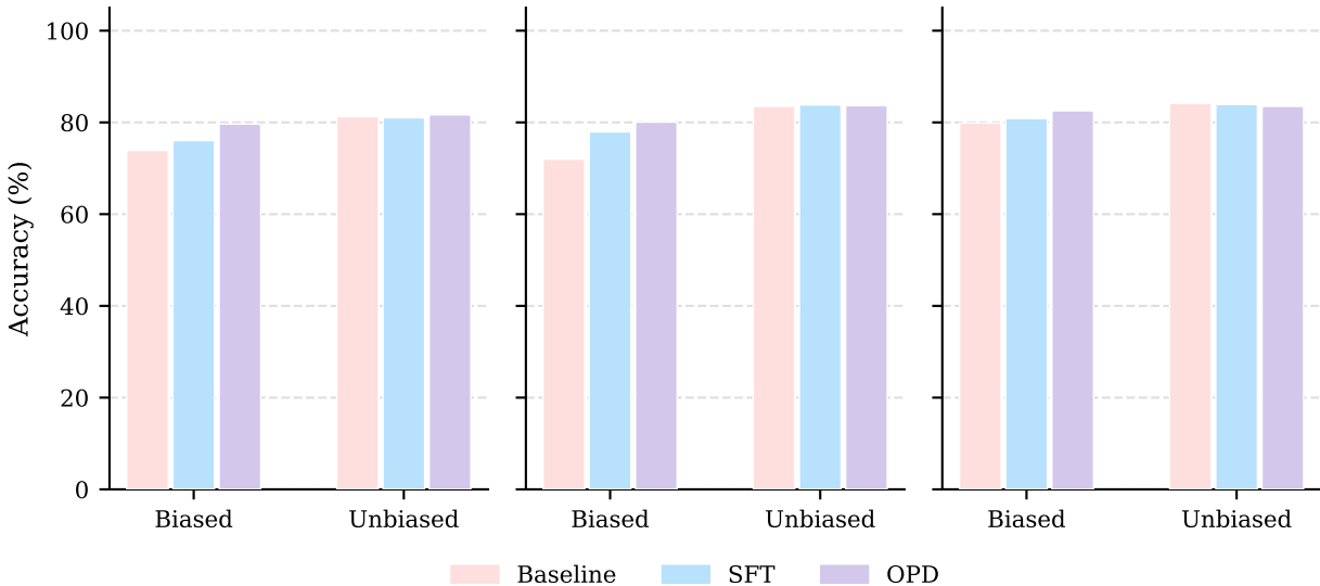
Qwen3-8B
