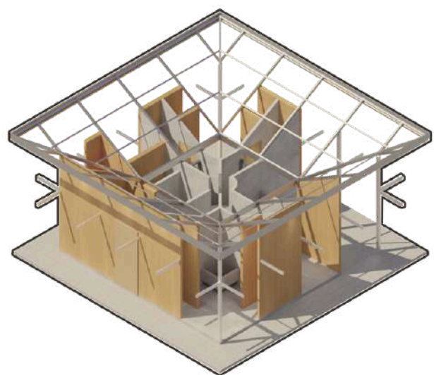
โครงสร้างหลังคาเหล็ก
