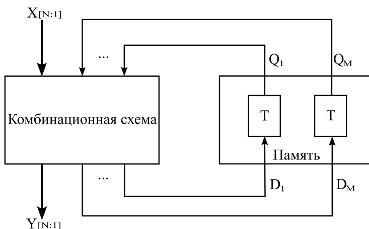
Рисунок 5.7 – Представление управляющей части нейронной сети в виде композиции памяти и комбинационной схемы
