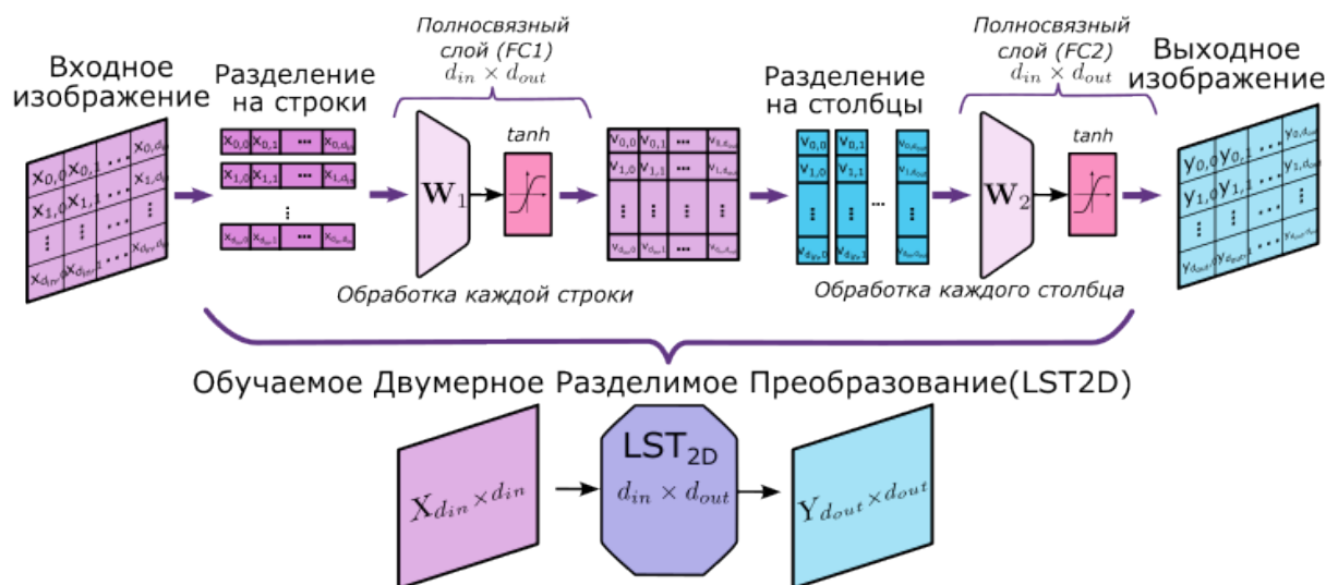
Рисунок 4.1 – Принцип работы LST2D
