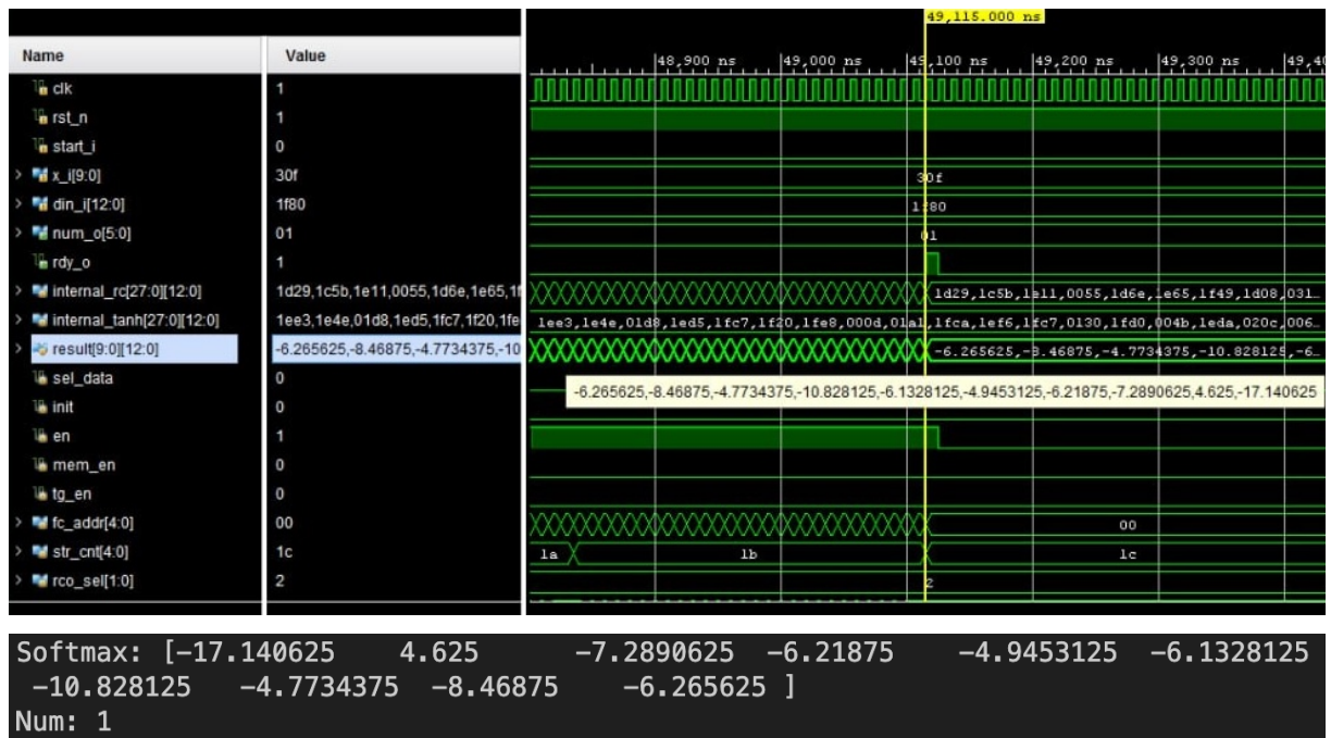
Рисунок 6.5 – Временная диаграмма нейронной сети и результат работы эталона на первом изображении
