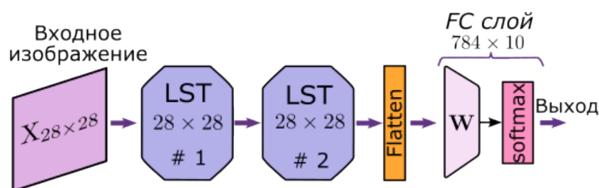
Рисунок 4.3 – Принцип работы LST-2
