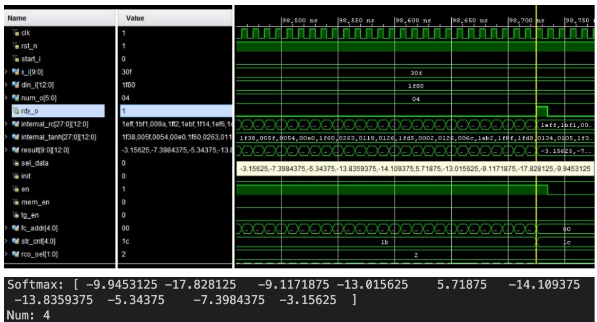
Рисунок 6.6 – Временная диаграмма нейронной сети и результат работы эталона на втором изображении
