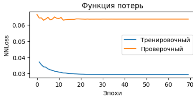
Рисунок 5.3 – Графики функции потерь на обучающем и тестовом наборе
