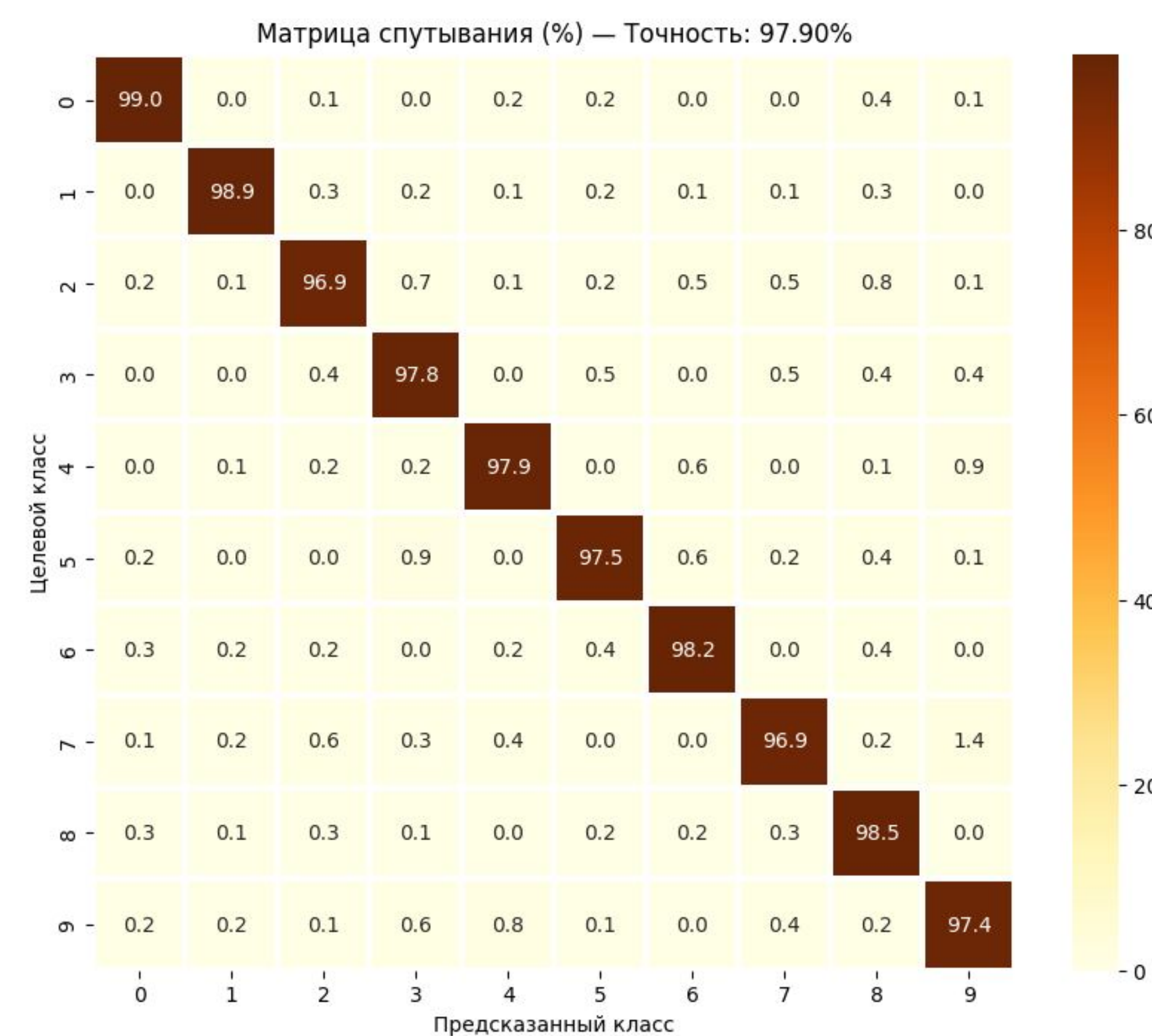
Матрица fixpoint
