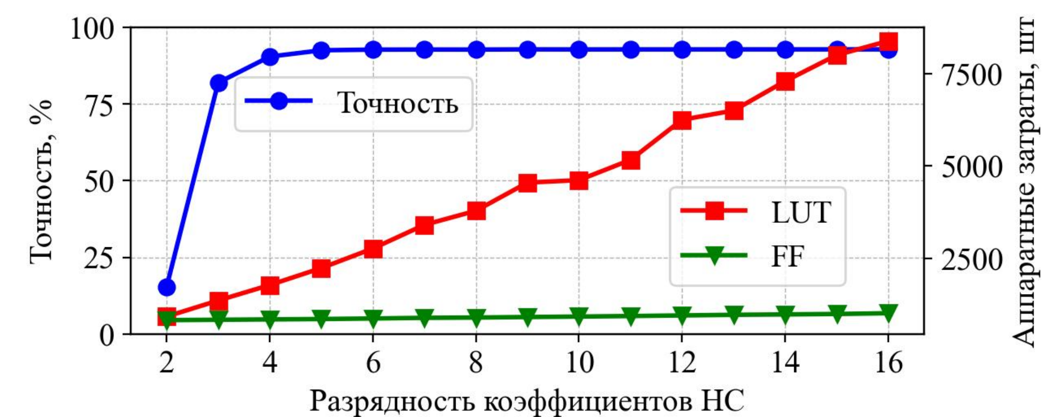
График точности
