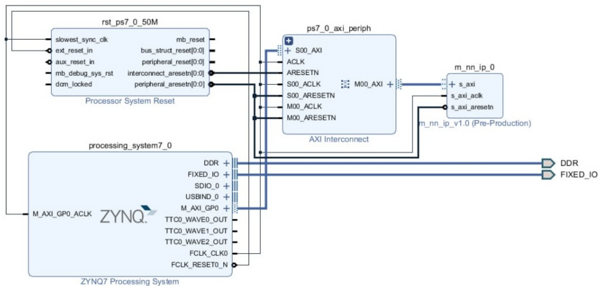
Рисунок 5.3 – Результирующий вид блочной диаграммы
