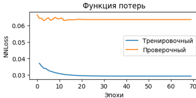
Рисунок 4.3 – Графики функции потерь на обучающем и тестовом наборе
