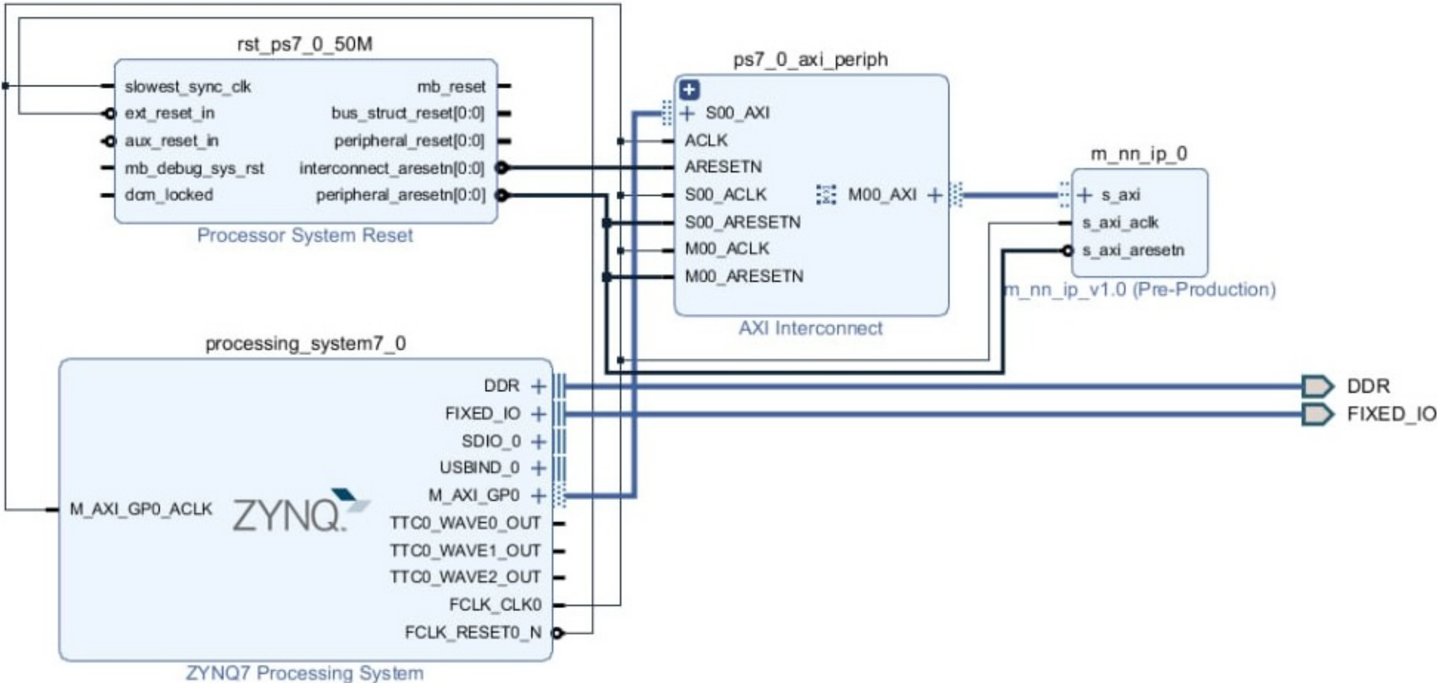
Блочная диаграмма
