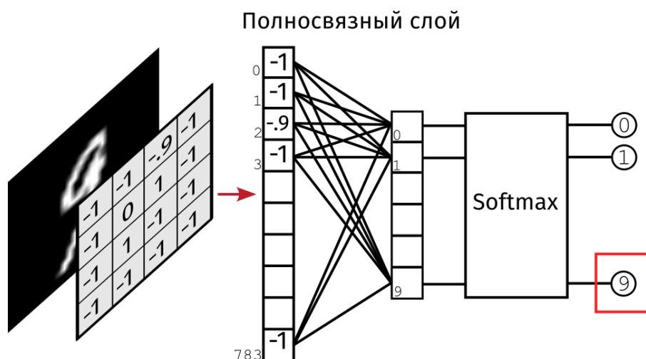
Рисунок 1.6 – Однослойной нейронной сети прямого распространения
