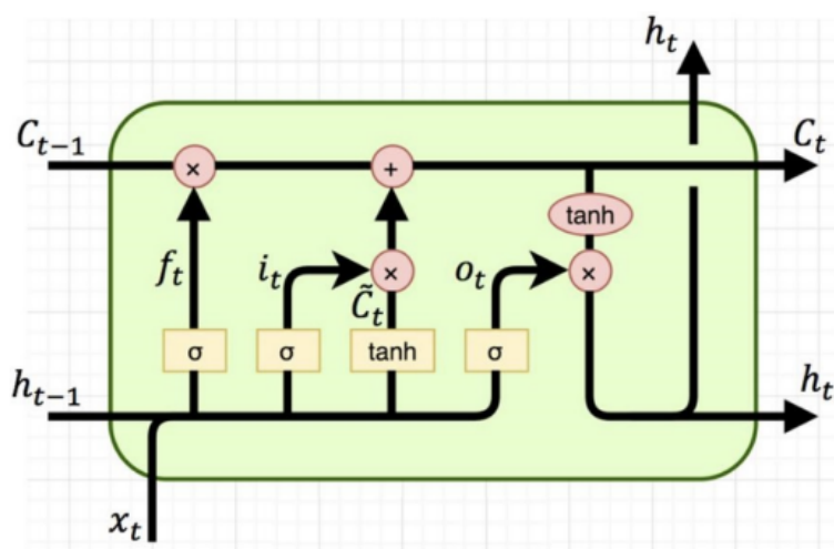
Рисунок 1.10 – Пример архитектуры LSTM
