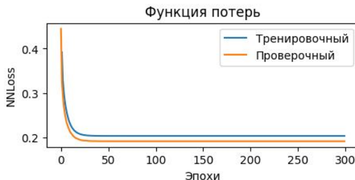
Рисунок 3.8 – Графики функции потерь на обучающем и тестовом наборе
