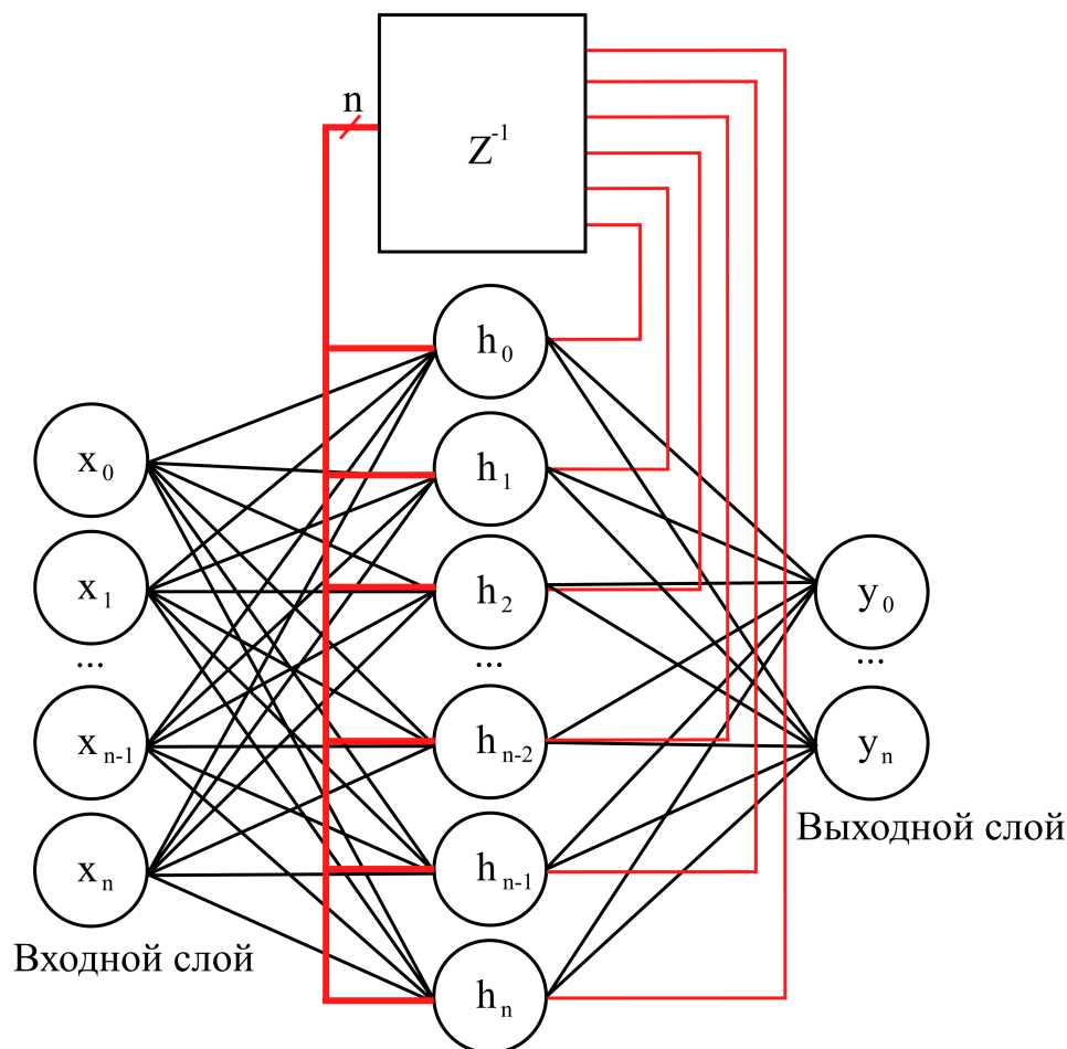
Рисунок 1.9 – Принцип работы рекуррентных нейронных сетей
