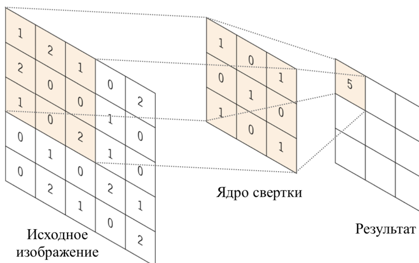
Рисунок 1.7 – Принцип работы сверточных нейронных сетей
