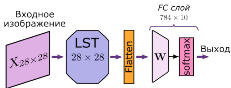
Рисунок 3.2 – Принцип работы LST-1
