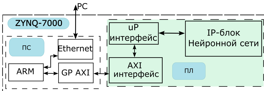
Рисунок 4.1 – Пример использования IP-блока нейронной сети
