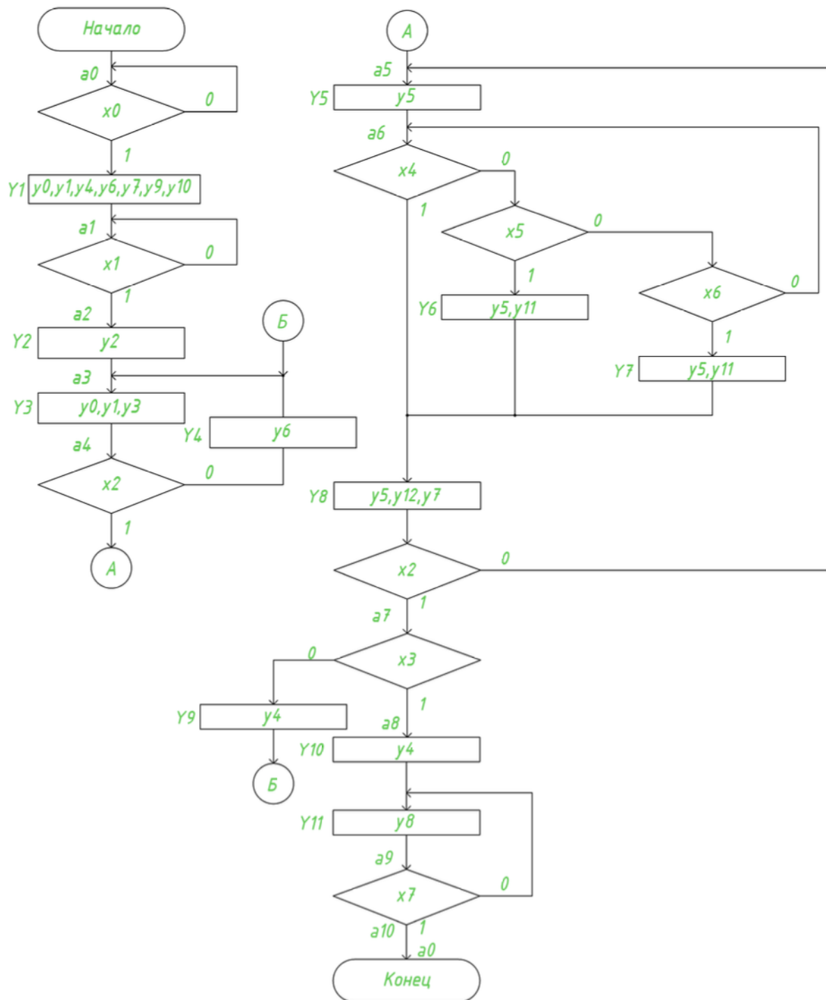
Рисунок 4.6 – Граф-схема алгоритма
