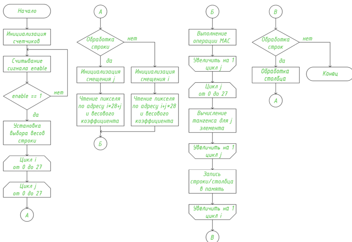
Рисунок 3.3 – Алгоритм работы LST2D слоя
