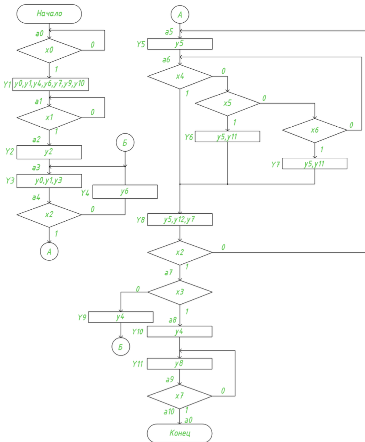
Рисунок 4.6 – Граф переходов
